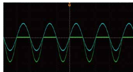
负半波整流
