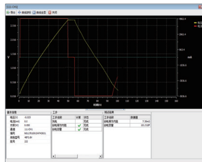
▲ 测试界面图
