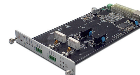
▲ N8070A CAN通讯卡
