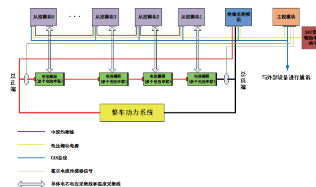
▲ 新能源汽车BMS示意图
