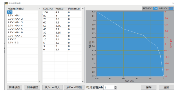
▲BMS测试系统软件电池模型界面
