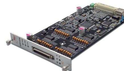
▲ N8030C PWM输出控制卡
