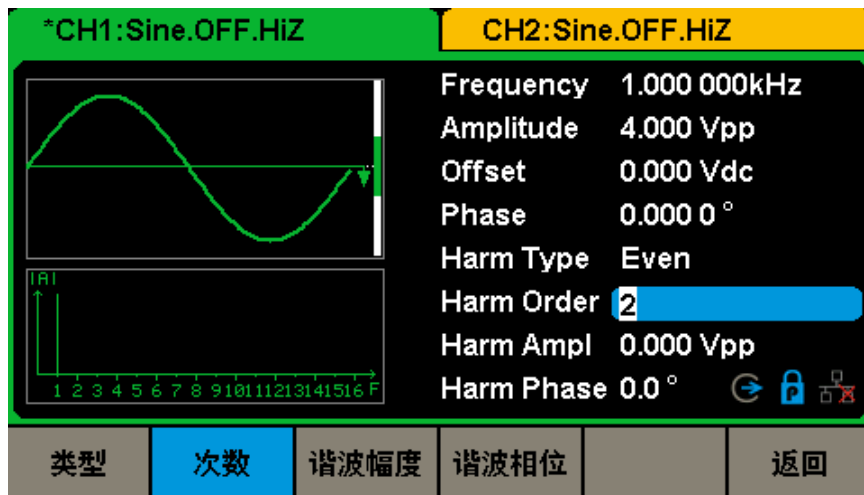
图 2-22 谐波设置界面
