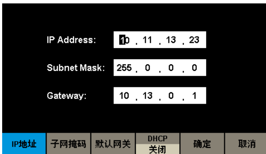
图 2-67 局域网参数设置界面
