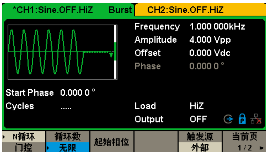
图 2-27 无限脉冲串
