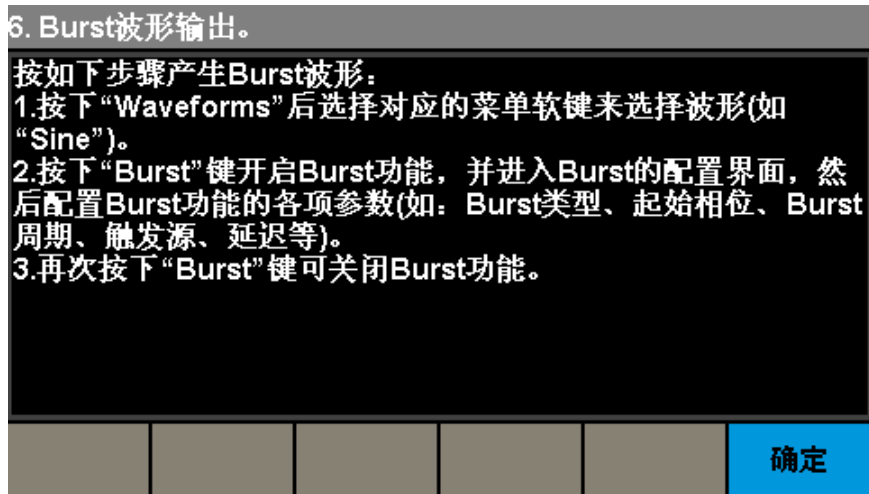
图 2-47 Burst 波形输出
