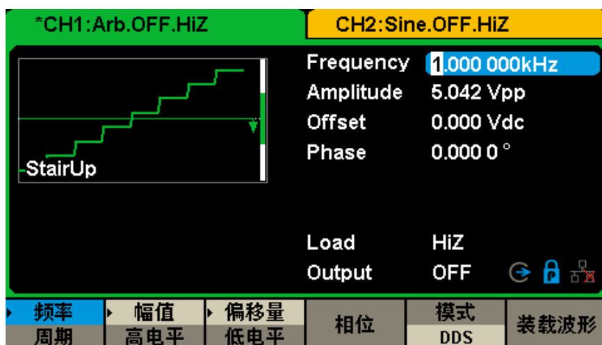
图 2-17 任意波 DDS 模式参数显示界面
