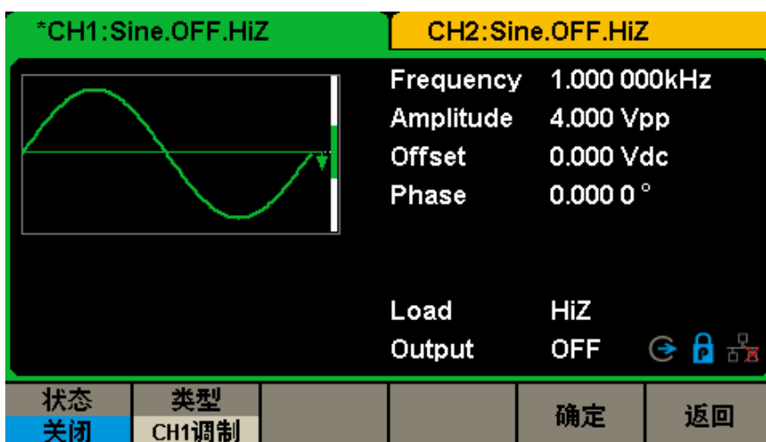
图 2-68 同步设置界面
