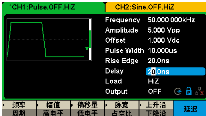
图 3-4 输出脉冲波
