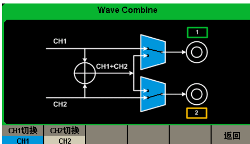
图 2-60 通道合并示意图
