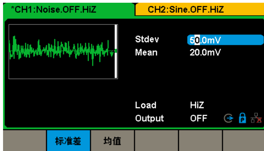
图 3-5 输出噪声
