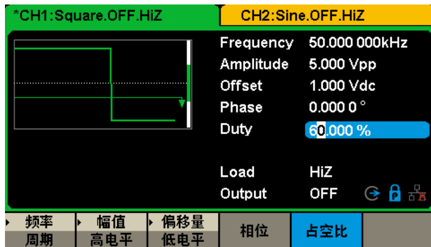
图 3-2 输出方波
