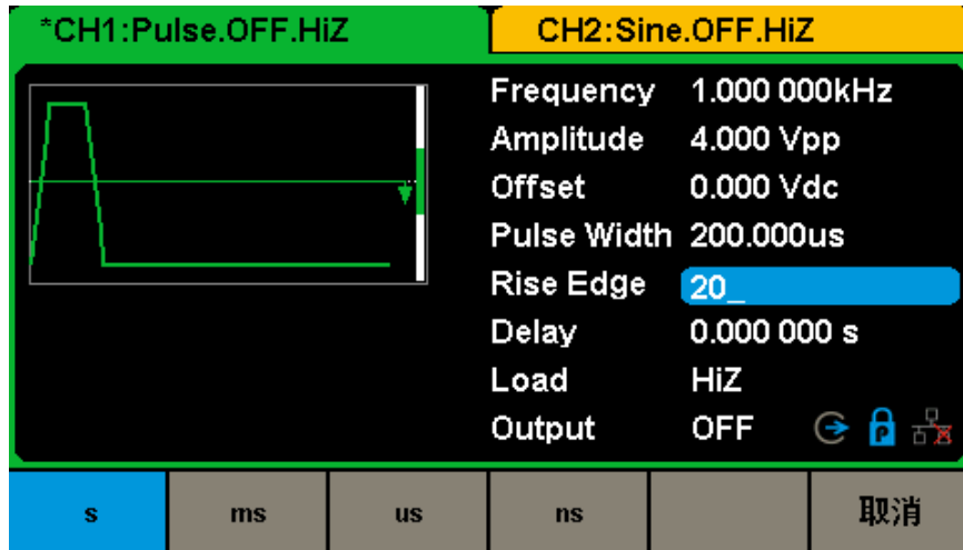
图 2-12 脉冲上升沿设置界面
