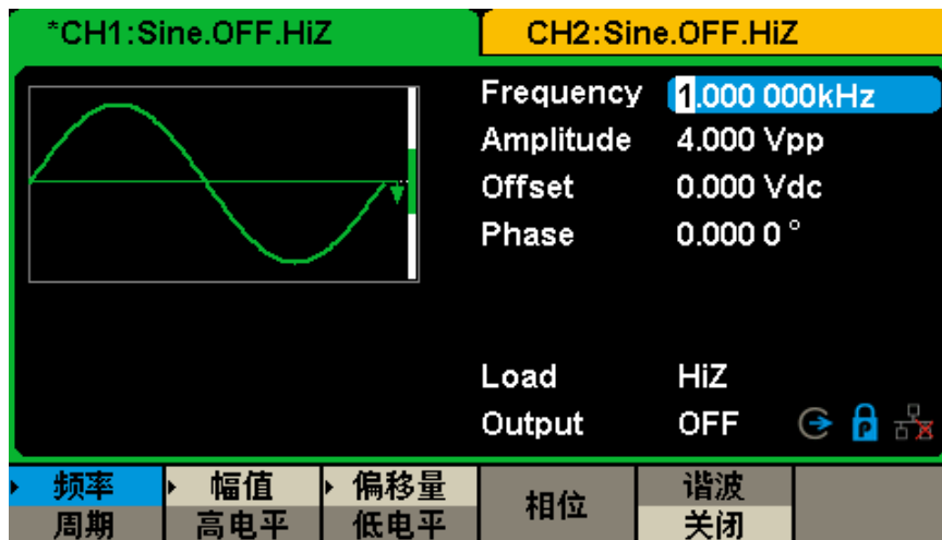
图 2-70 相位锁定模式
