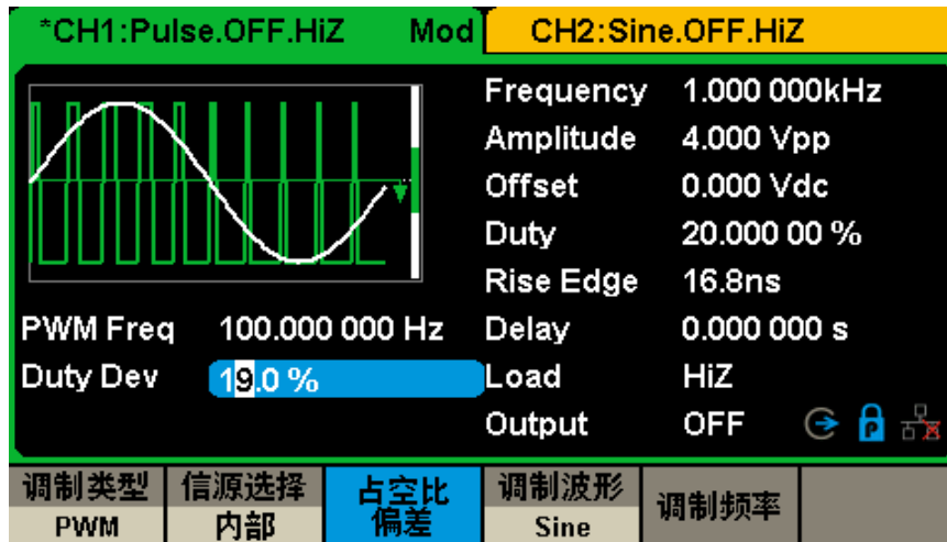
图 2-24 设置 PWM 占空比偏差
