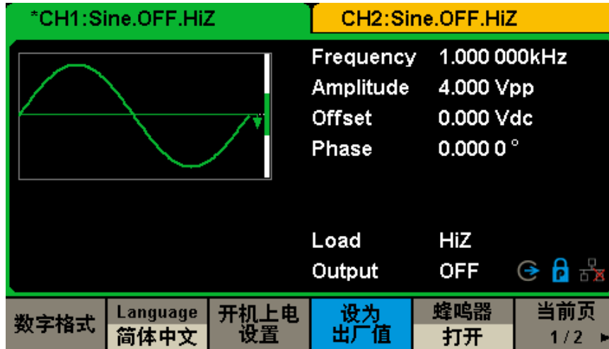
图 2-32 系统设置操作界面（当前页 1/2）
