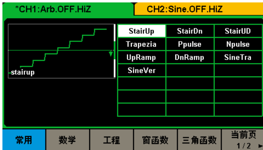
图 2-20 内建的任意波
