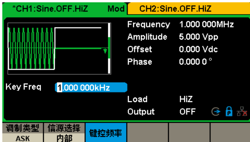
图 3-13 输出 ASK 调制波形
