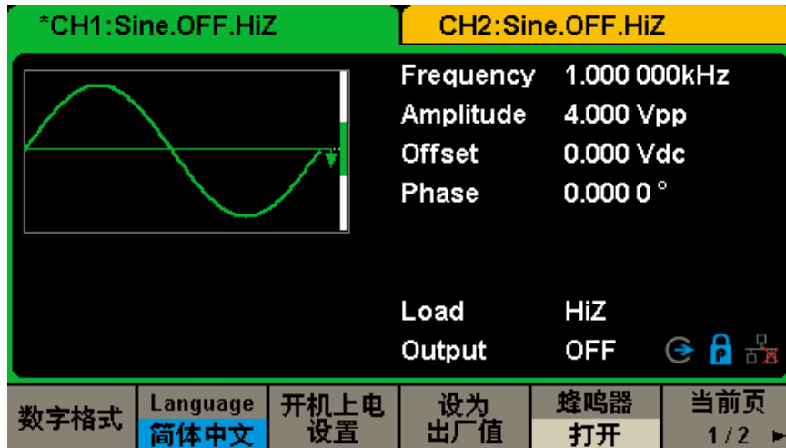
图 2-37 中文显示界面
