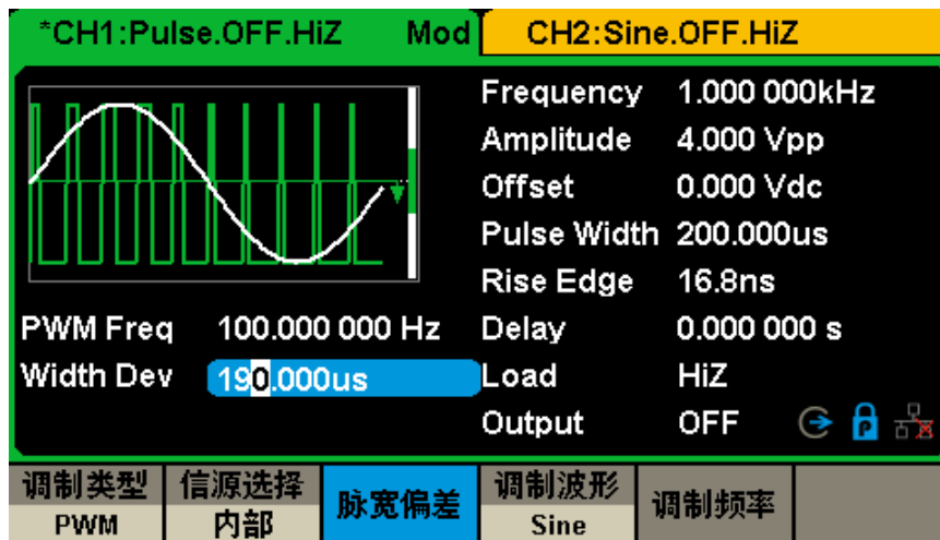
图 2-23 设置 PWM 脉宽偏差
