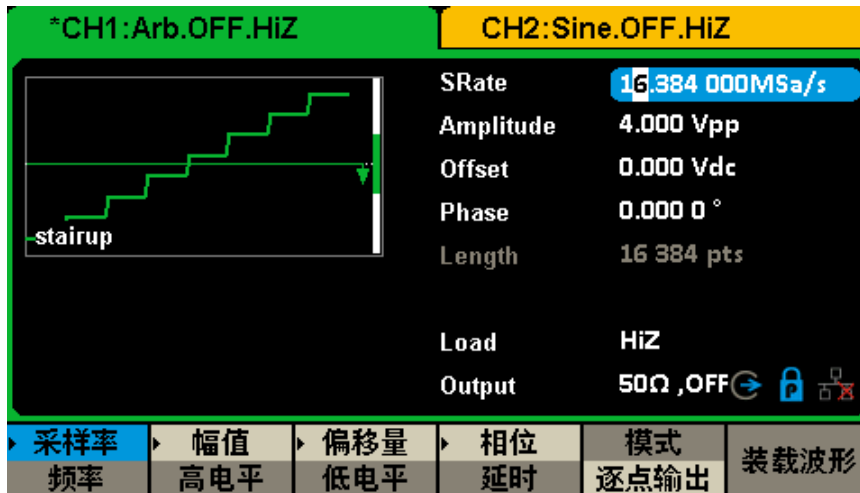
图 2-18 任意波逐点输出模式显示界面
