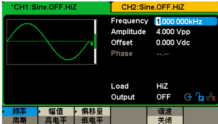
图 2-71 独立通道模式
