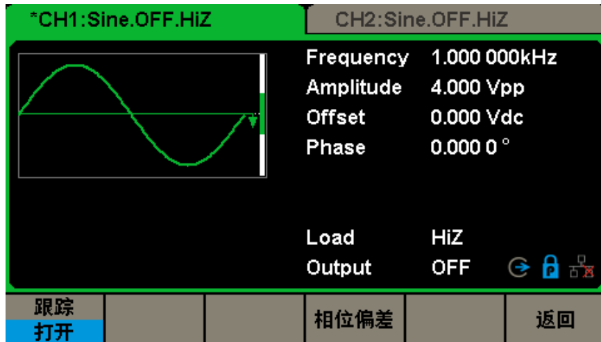
图2-63 跟踪功能界面
