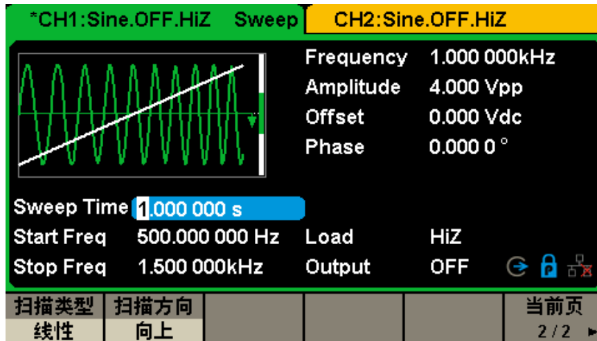
图 2-25 Sweep 线性扫频
