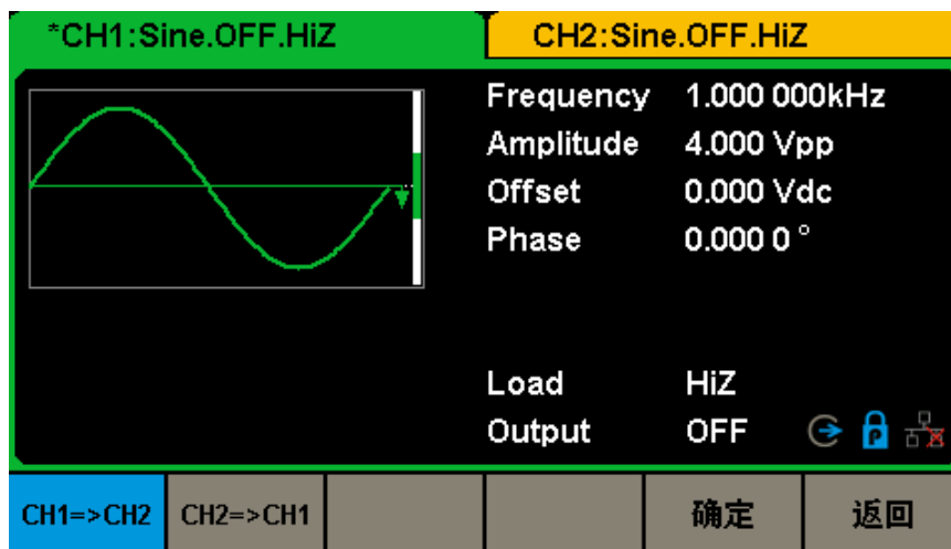
图 2-61 通道复制菜单
