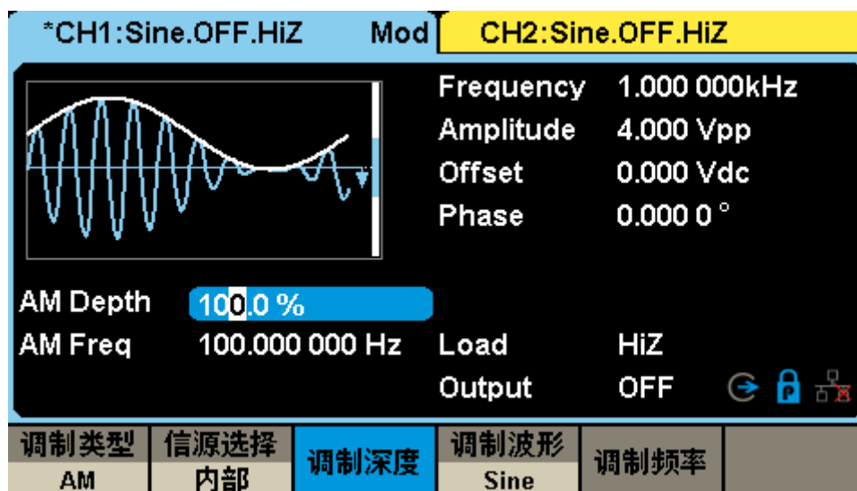
图 1-18 调制界面
