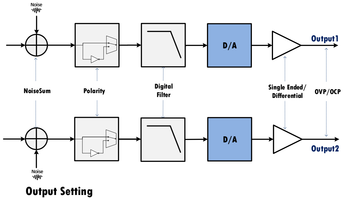
图 13.1 输出设置原理框图
