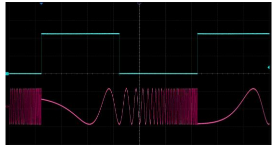
对数扫频结果
