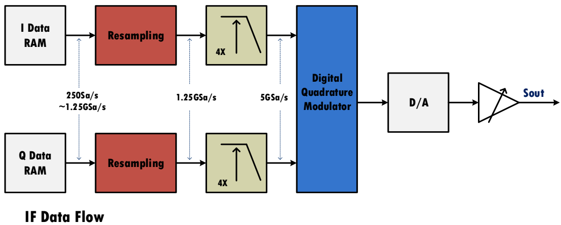
图 9.5 中频信号模式
