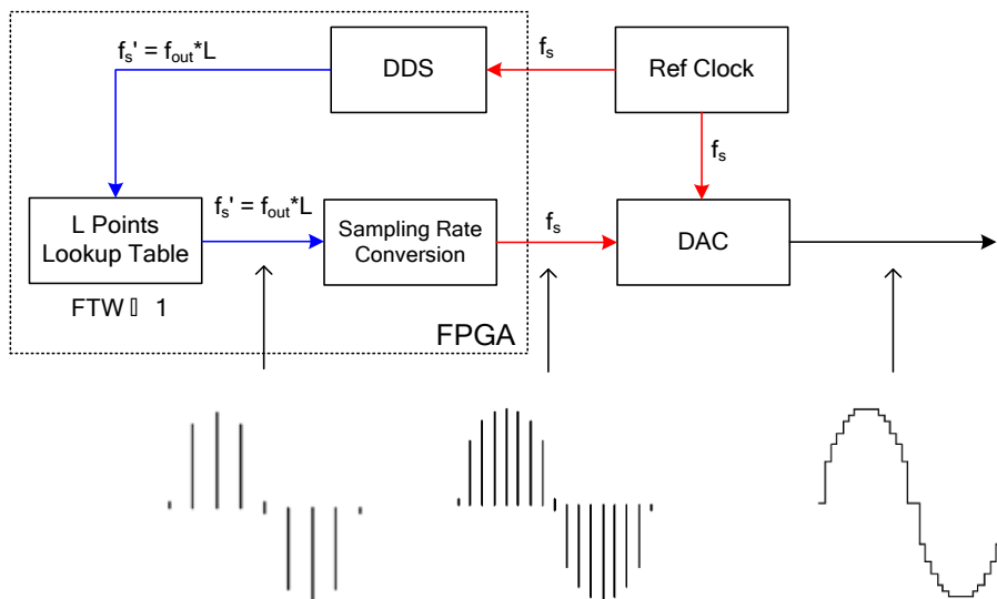
图 9.2 TrueArb 技术原理框图
