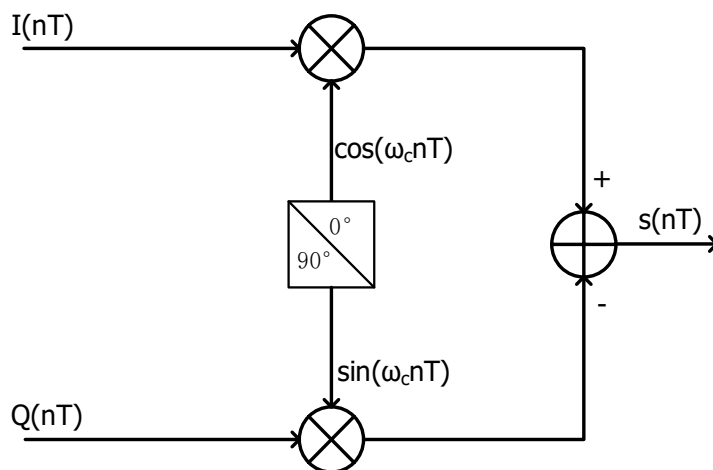
图 9.6 正交调制器的原理框图
