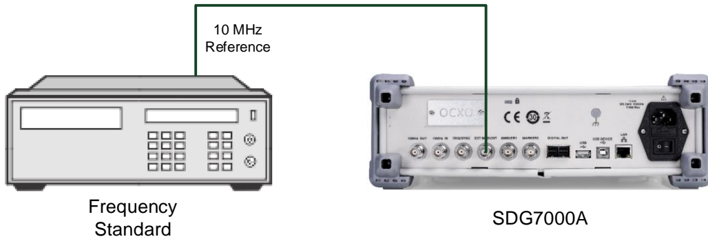
图 17.2 时基校准环境
