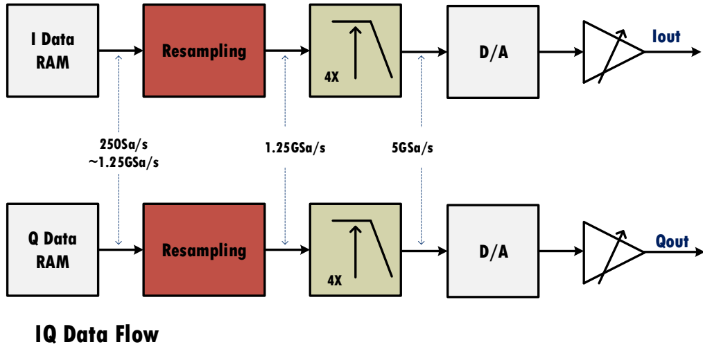
图 9.4 基带 I/Q 模式
