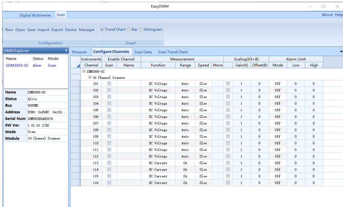
图 2-42 采样通道配置
