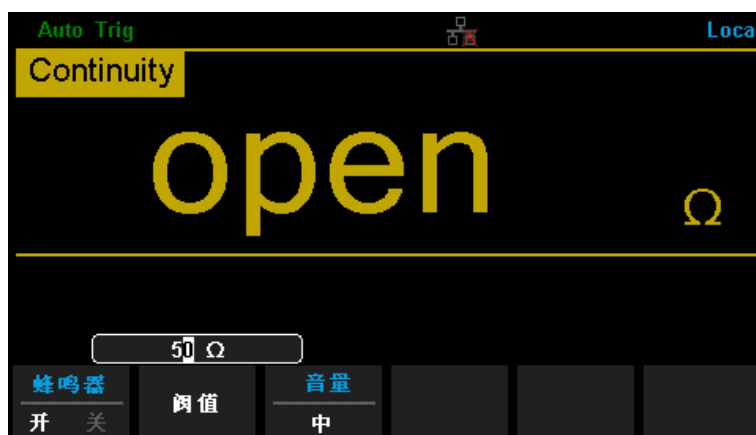
图 2-48 设置短路电阻
