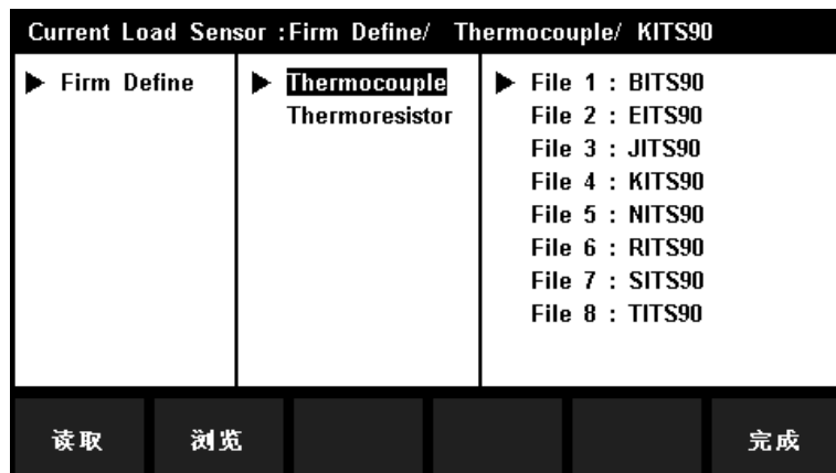
图 3-8 选择热电偶的类型
