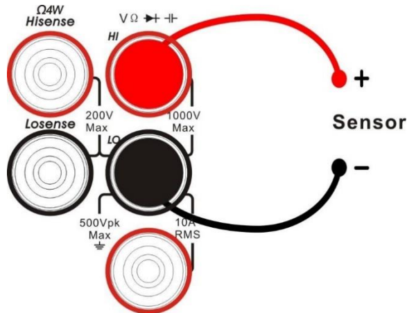
图 2-28 温度测量示意图
