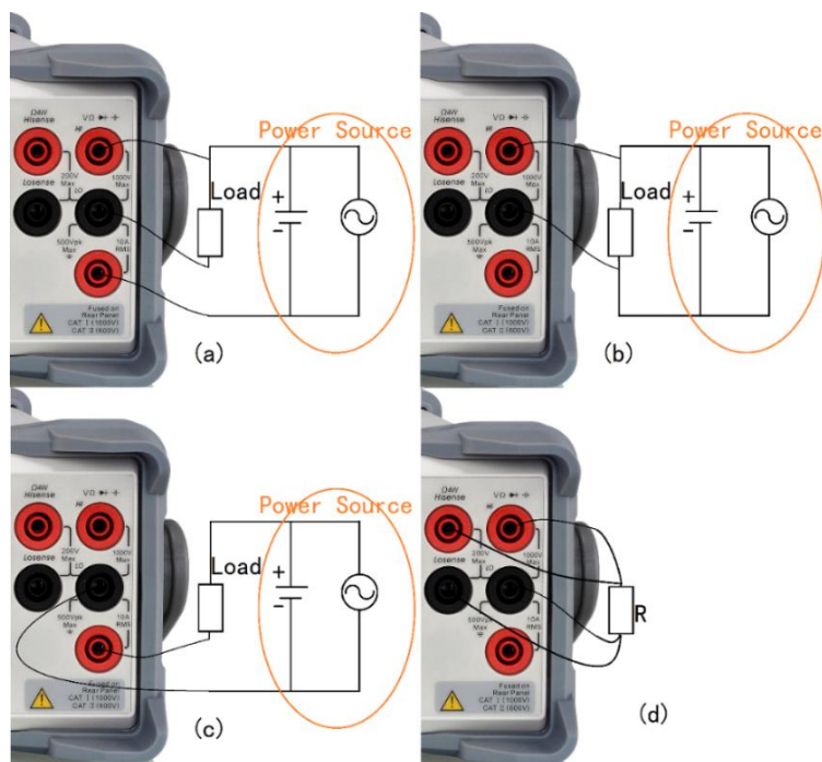
图 2-50 接线示例
