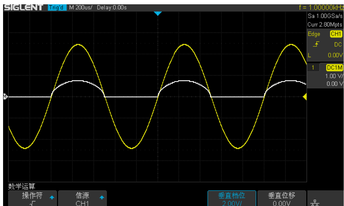
图 100 平方根运算
