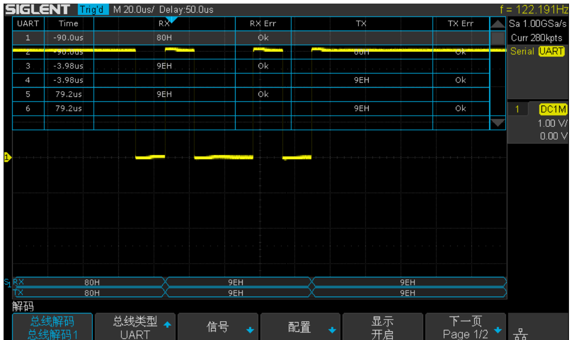
图 71 UART 解码图
