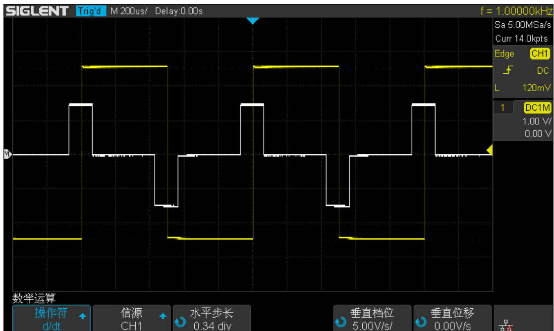
图 97 微分运算
