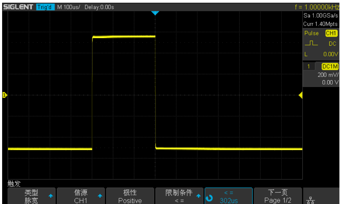
图 40 脉宽触发
