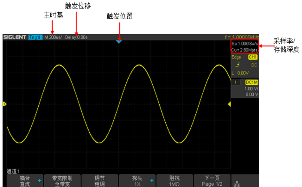
图 17 水平控制
