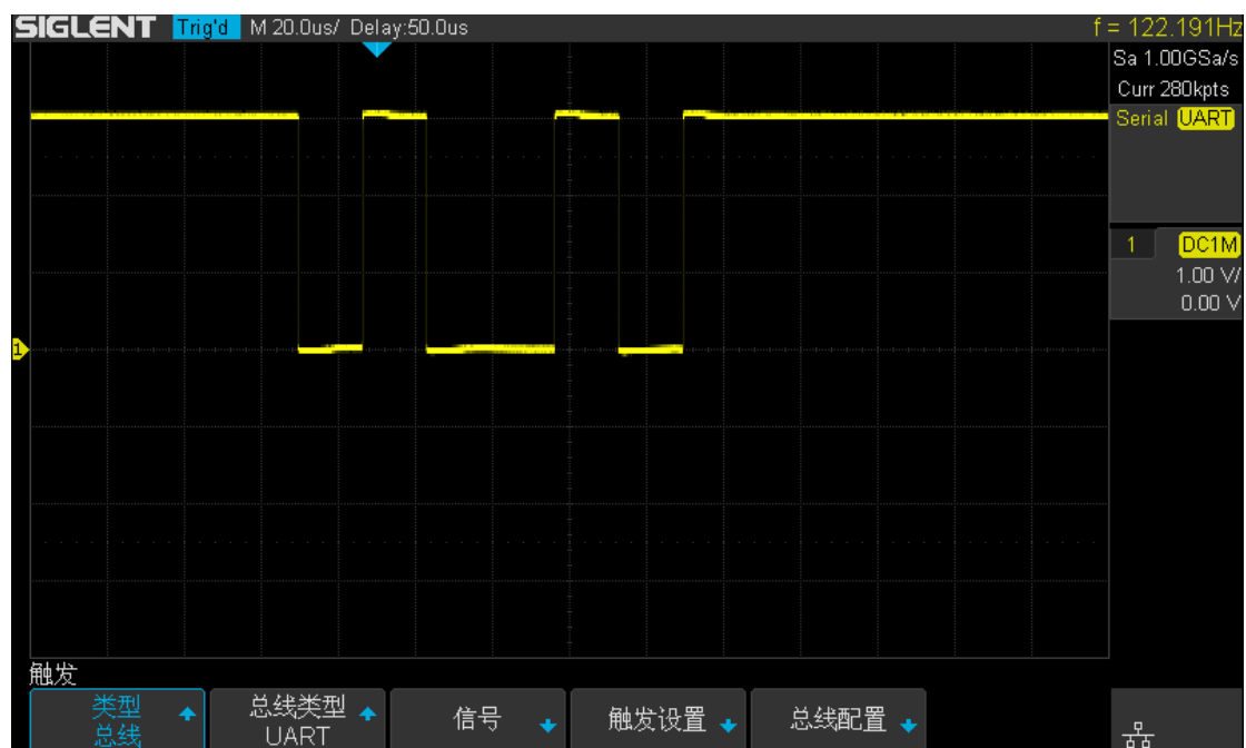
图 69 UART 触发
