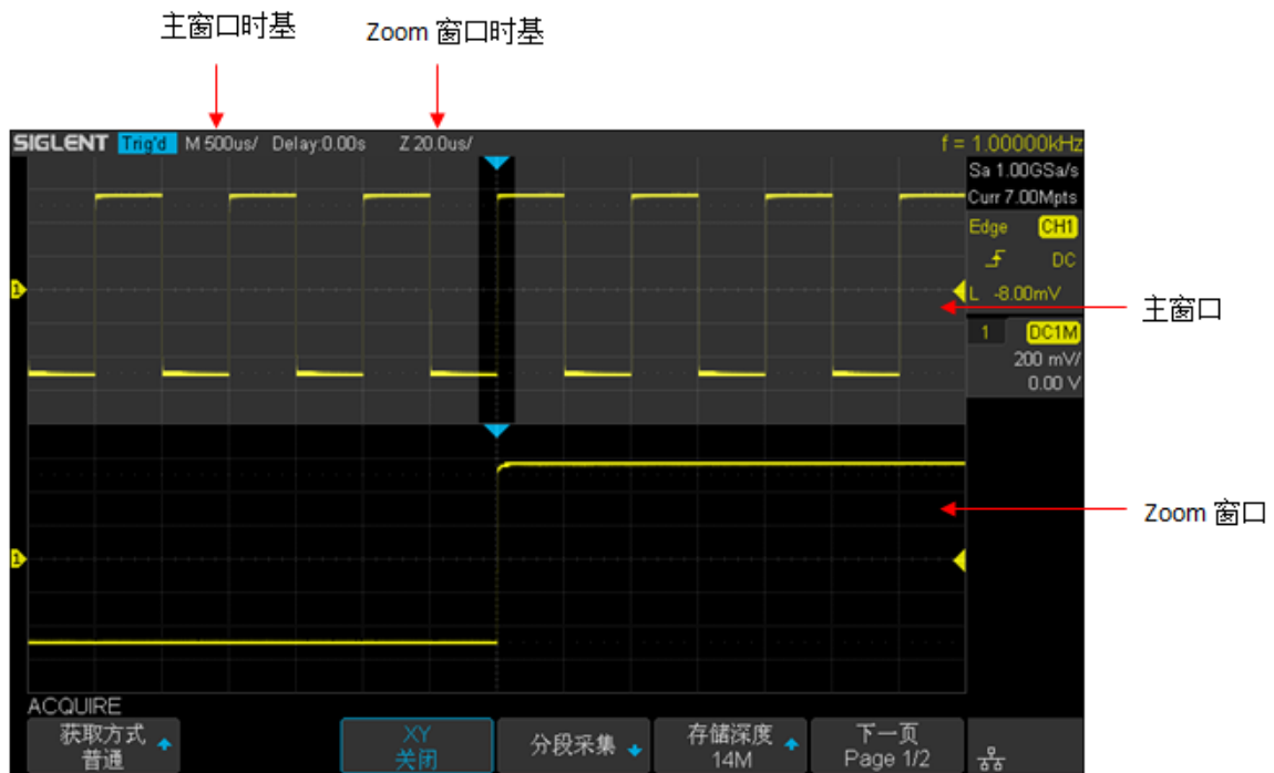
图 22 分屏缩放
