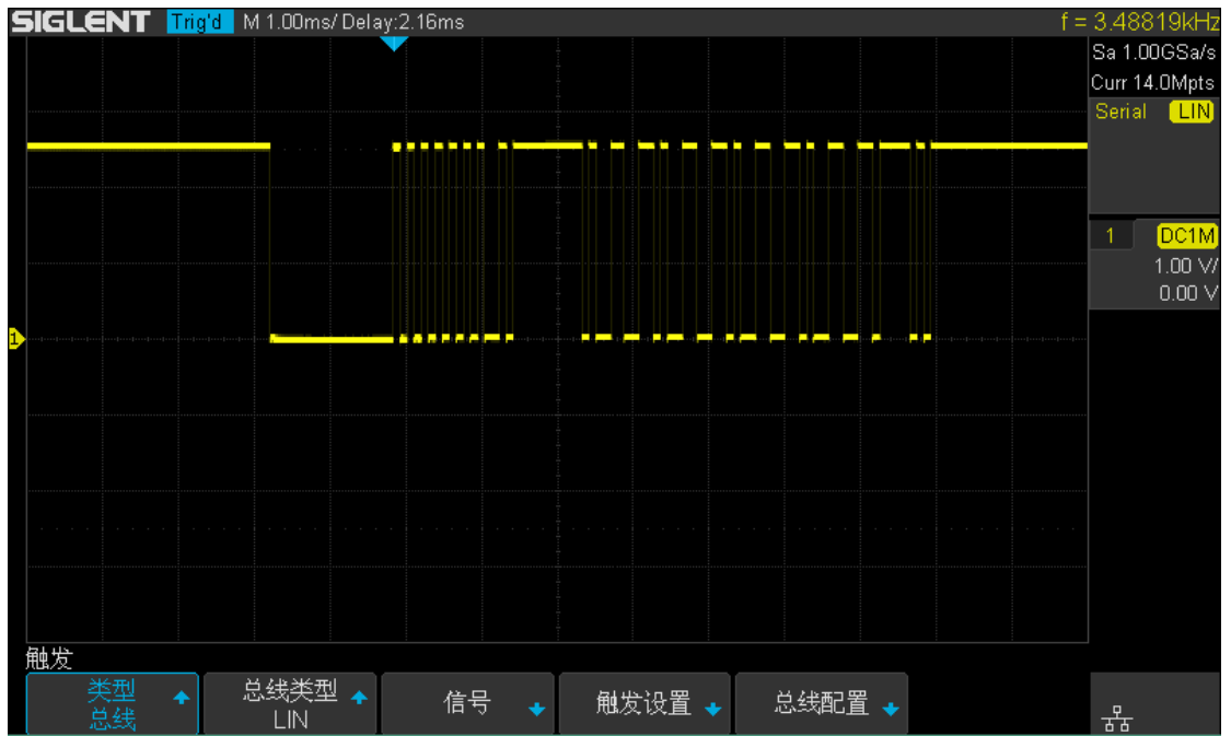
图 81 LIN 触发
