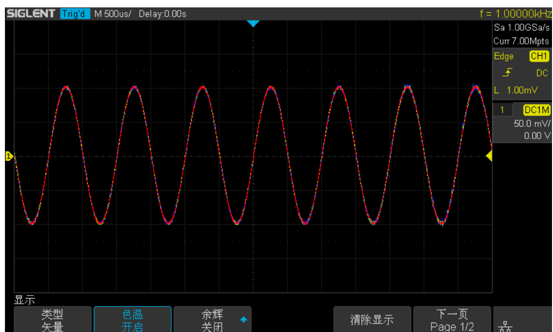
图 115 色温开启
