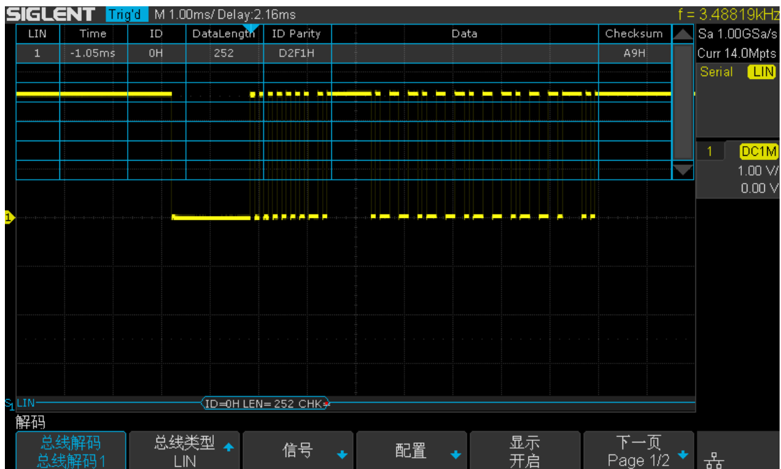
图 82 LIN 解码
