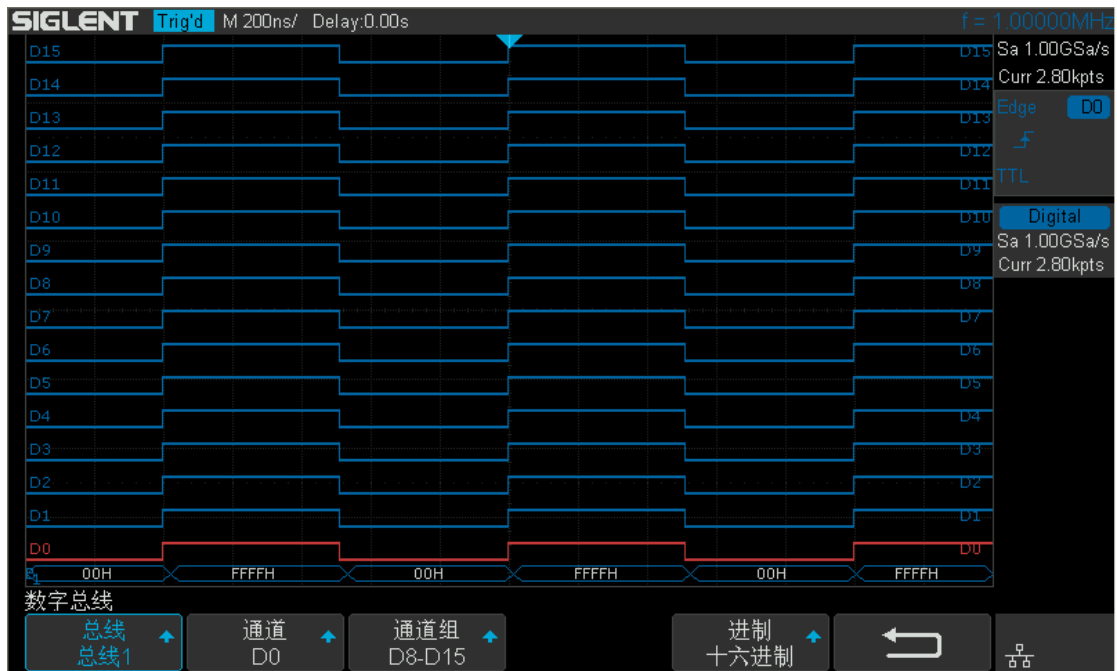
图 126 数字总线
