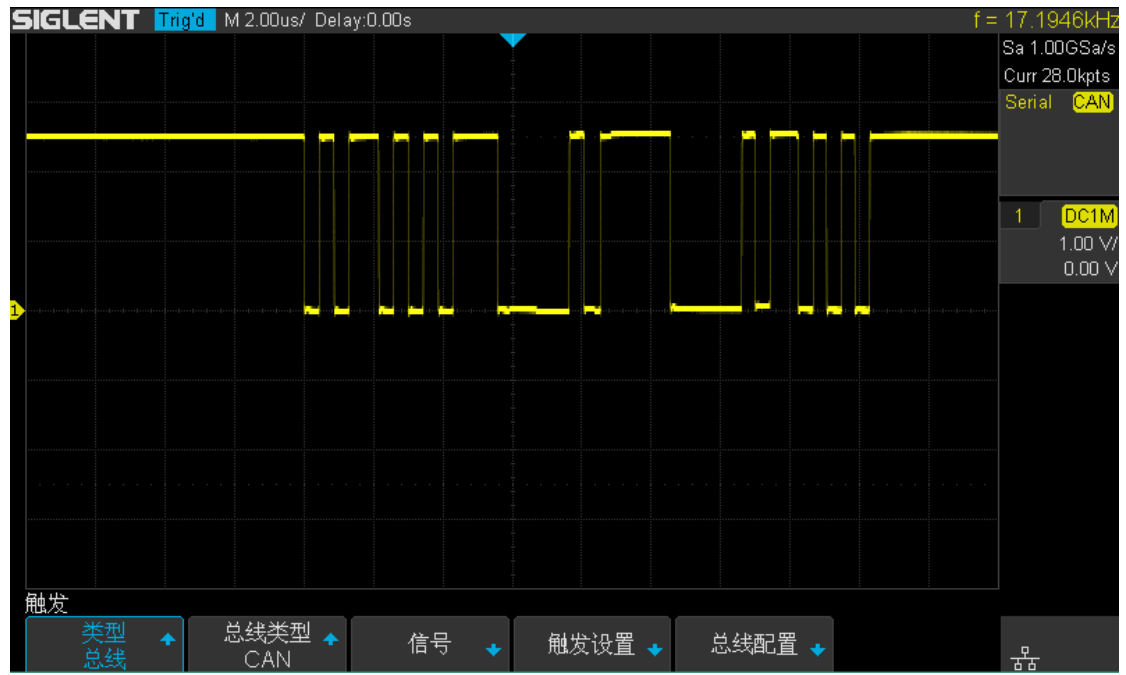
图 76 CAN 触发
