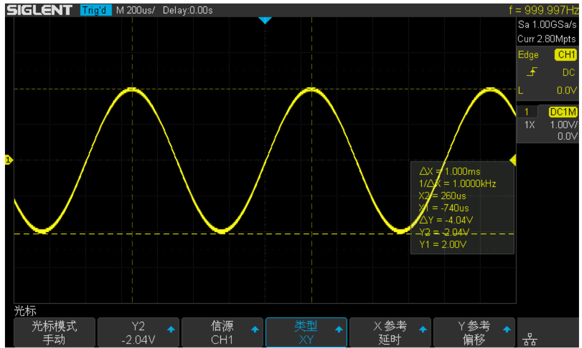
图 101 光标测量
