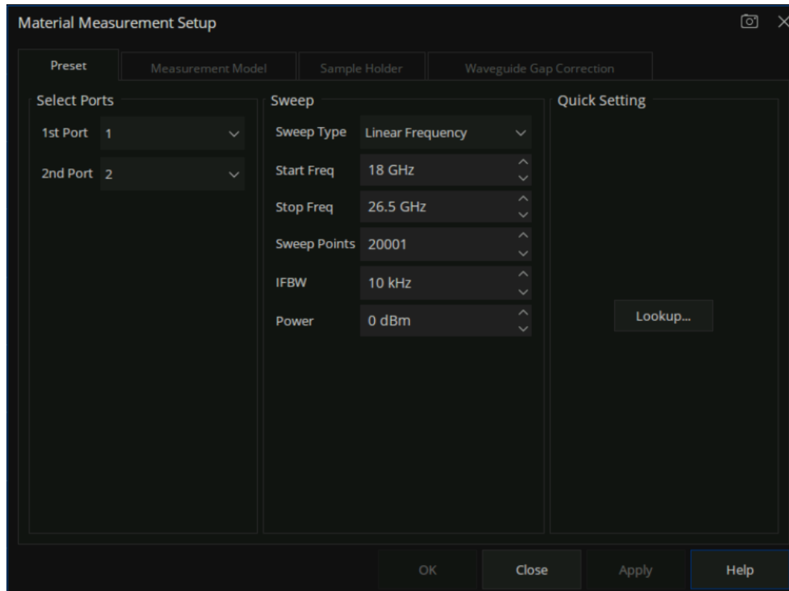
图 15-4 Preset 选项卡
