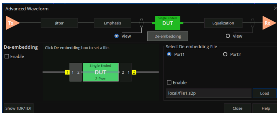
图 10-17 TDR 去嵌入设置
