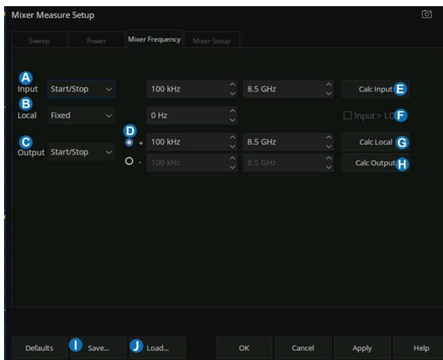
图 13-5 Mixer Frequency 选项卡
