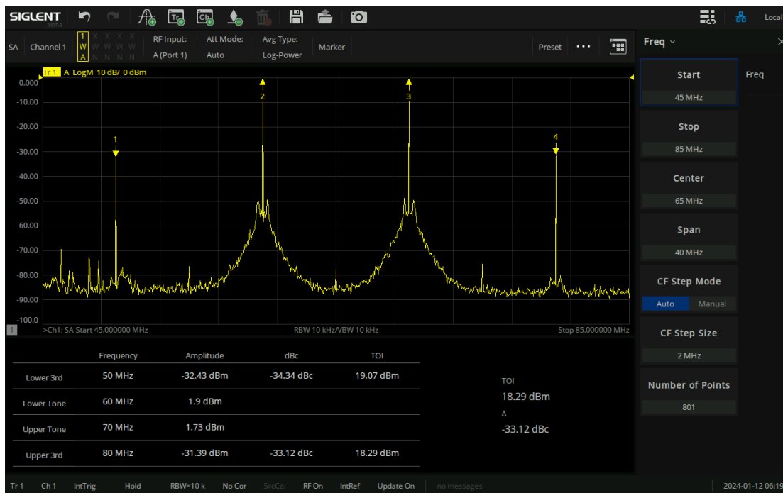
图 11-16 三阶交调测量界面
