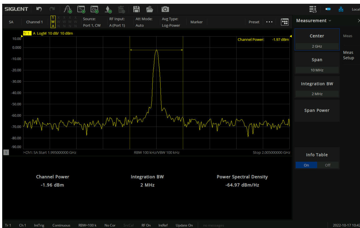
图 11-11-13 Channel Power 界面
