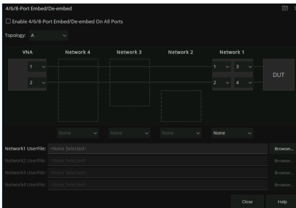
图 7-11 去嵌入界面
