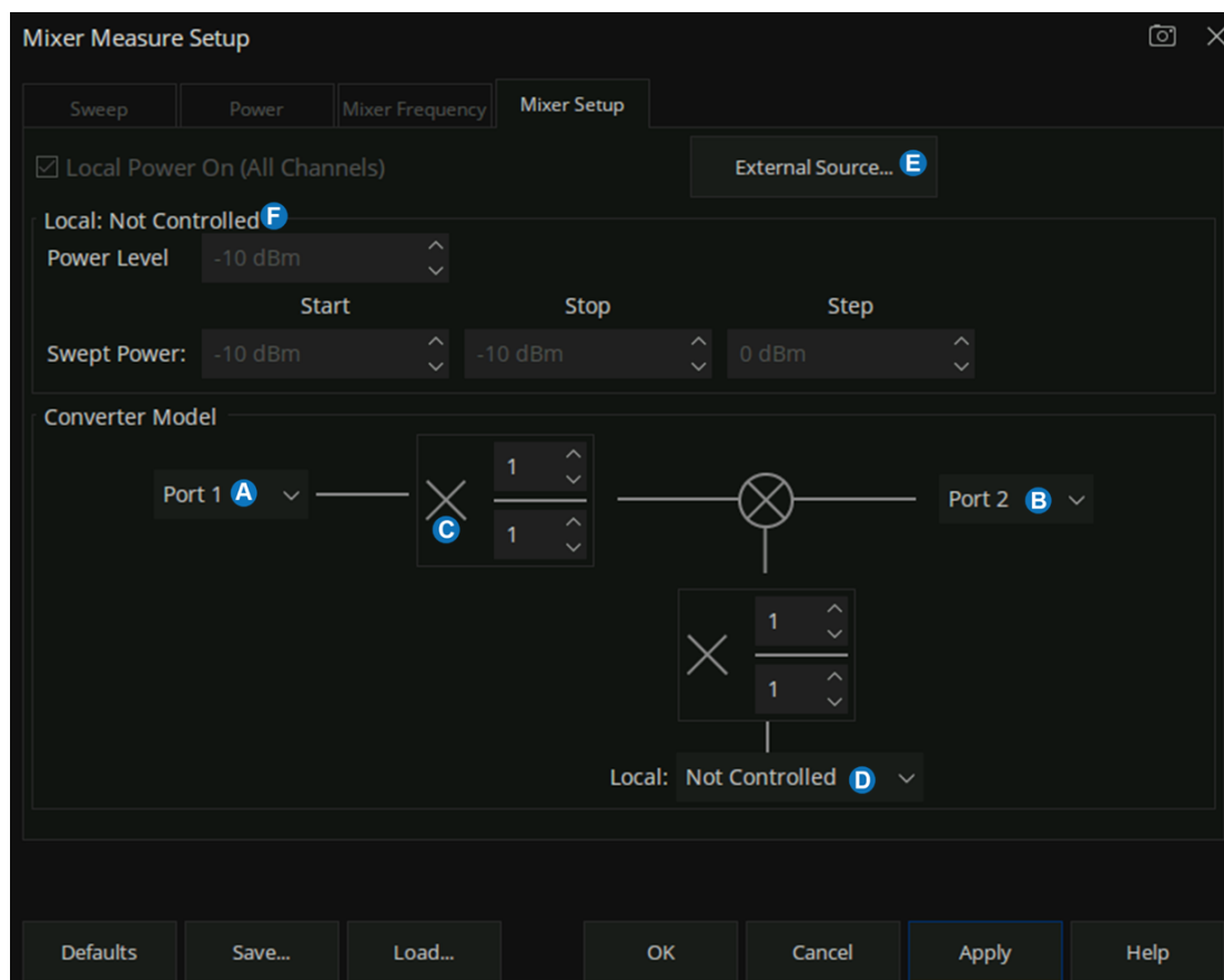
图 13-7 Mixer Setup 选项卡
