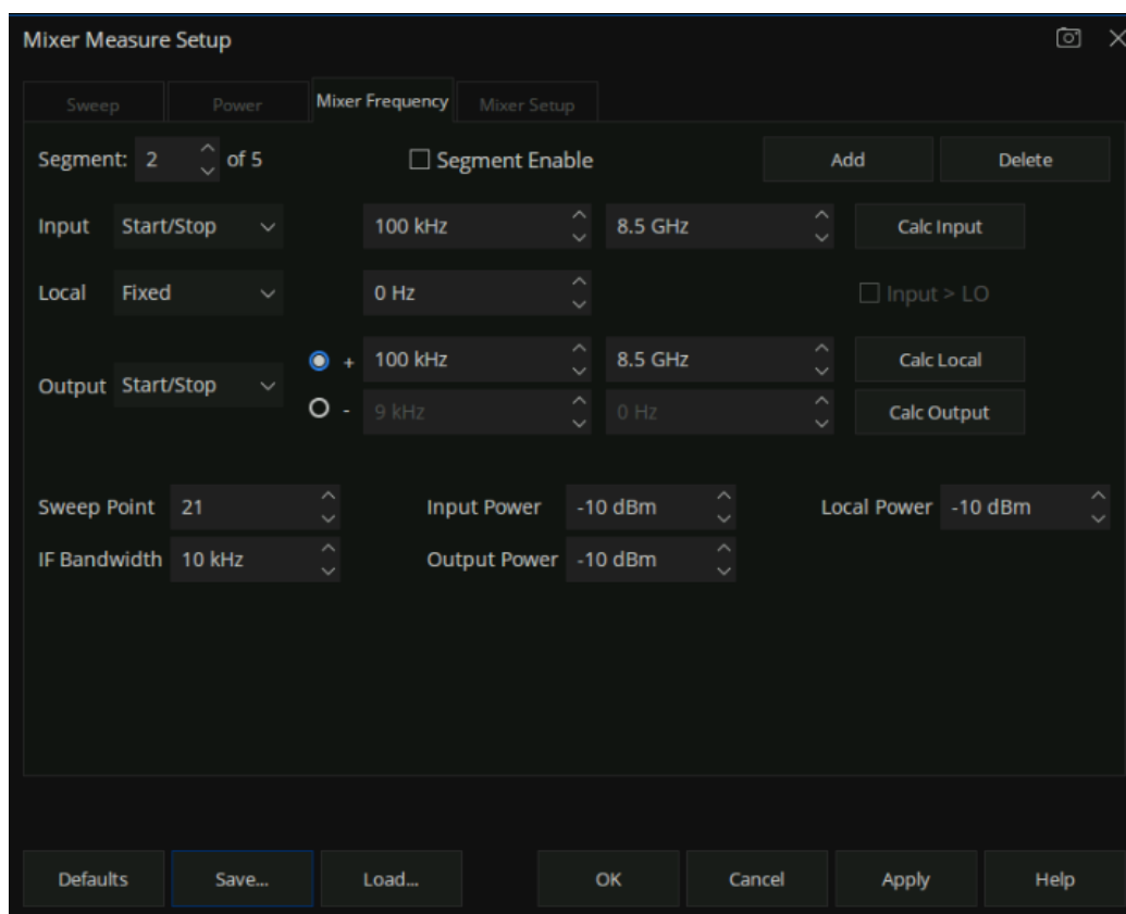
图 13-6 段扫描 Mixer Frequency 选项卡
