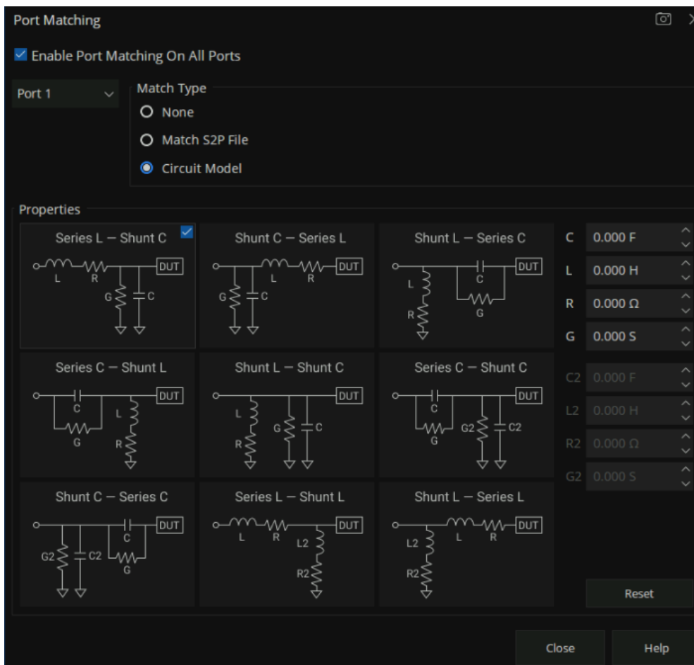
图 7-8 端口匹配
