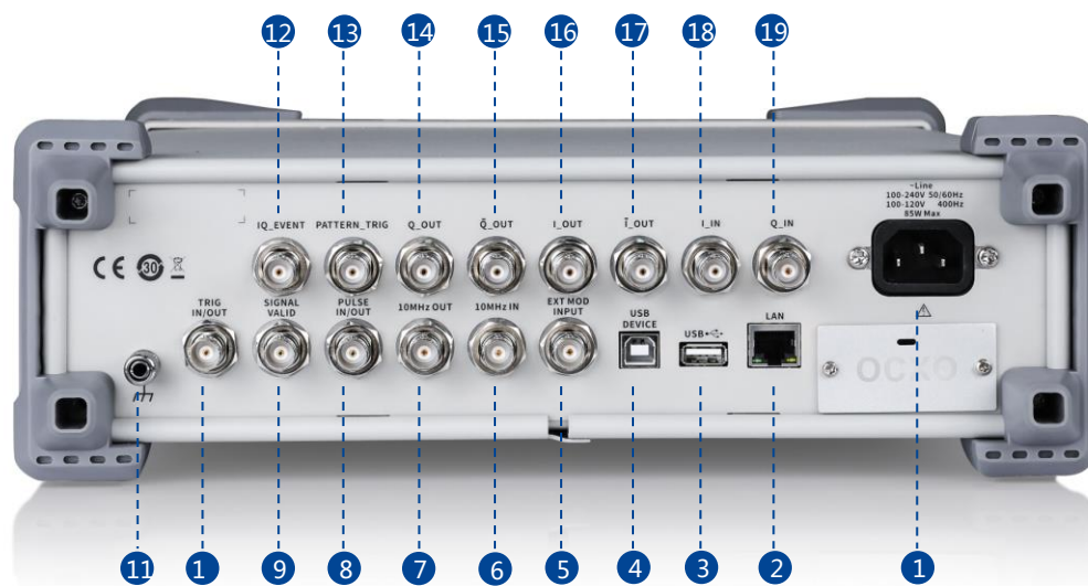
图 1-10 后面板
