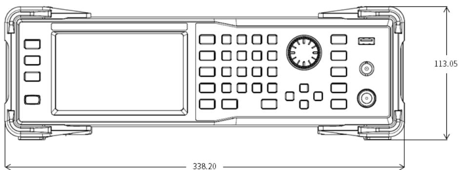
图 1-1 正视图
