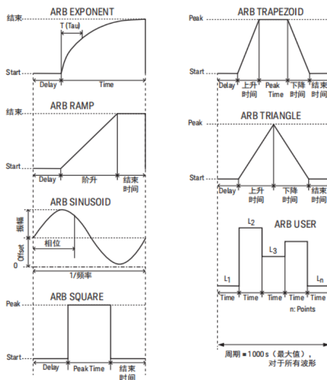
各种任意波形输出
