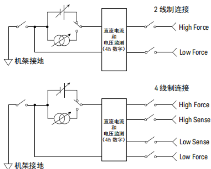
图 3-1 简化的电源电路图。
