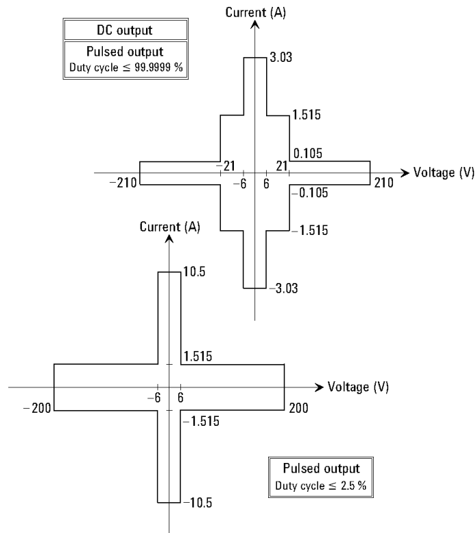
图 3-2 输出量程
