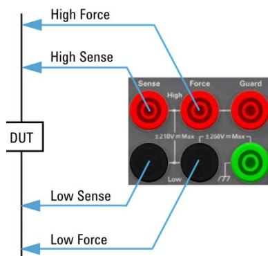
图 5-3 四线制连接
