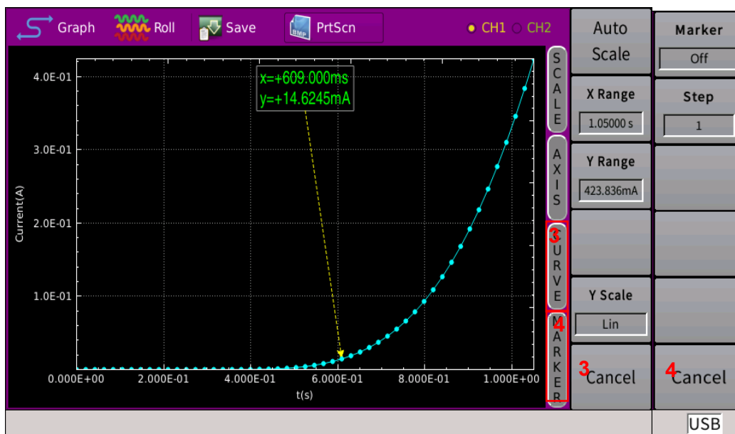
图 4-23 Roll 显示页面
