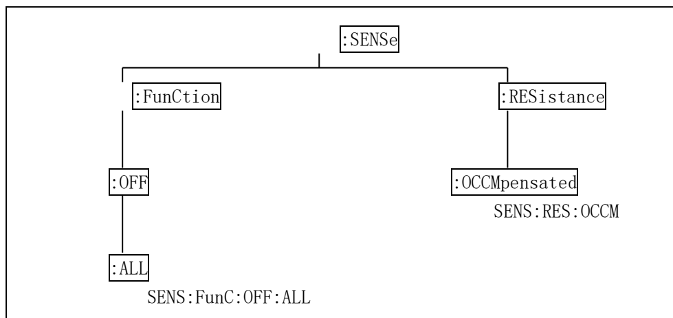
图 6-1 命令树层次
