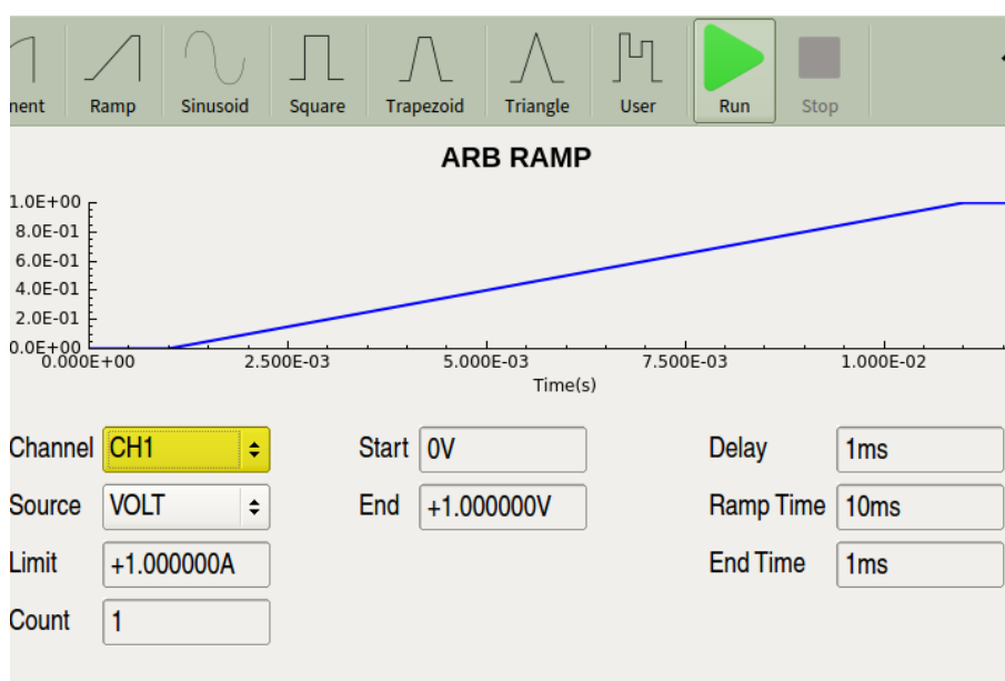
图 4-27 斜波波形输出
