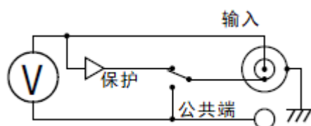
图 4-4 电压表简化电路图
