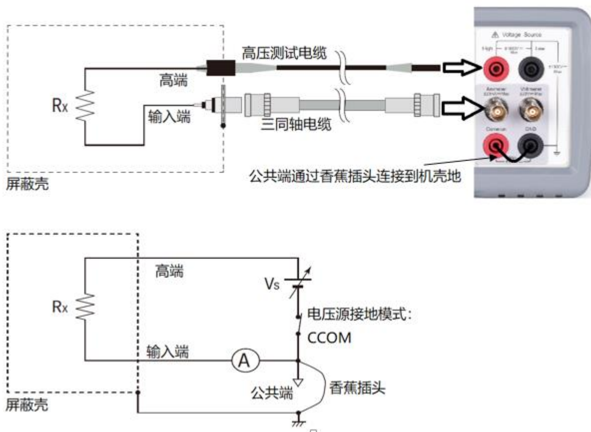
图 4-6 接地设备的测量
