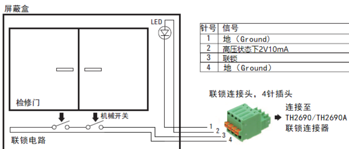
图 4-9 联锁电路
