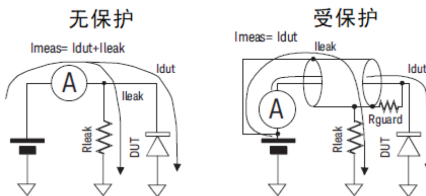
图 4-3 保护技术
