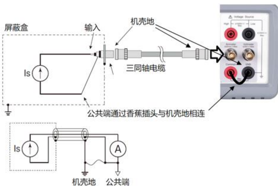
图 4-2 典型的接地的电流测量连接方式
