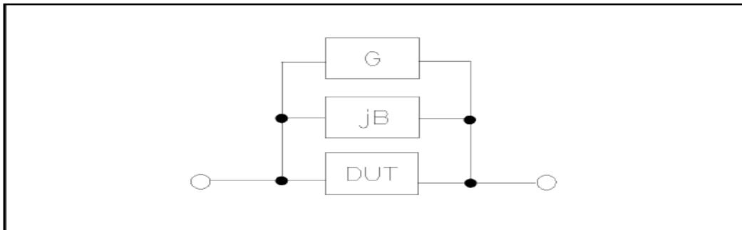
图 3-1 杂散导纳
