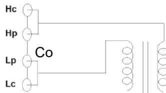
图 5—21 变压器绕组间电容测量 测试线可使用 TH26011。
