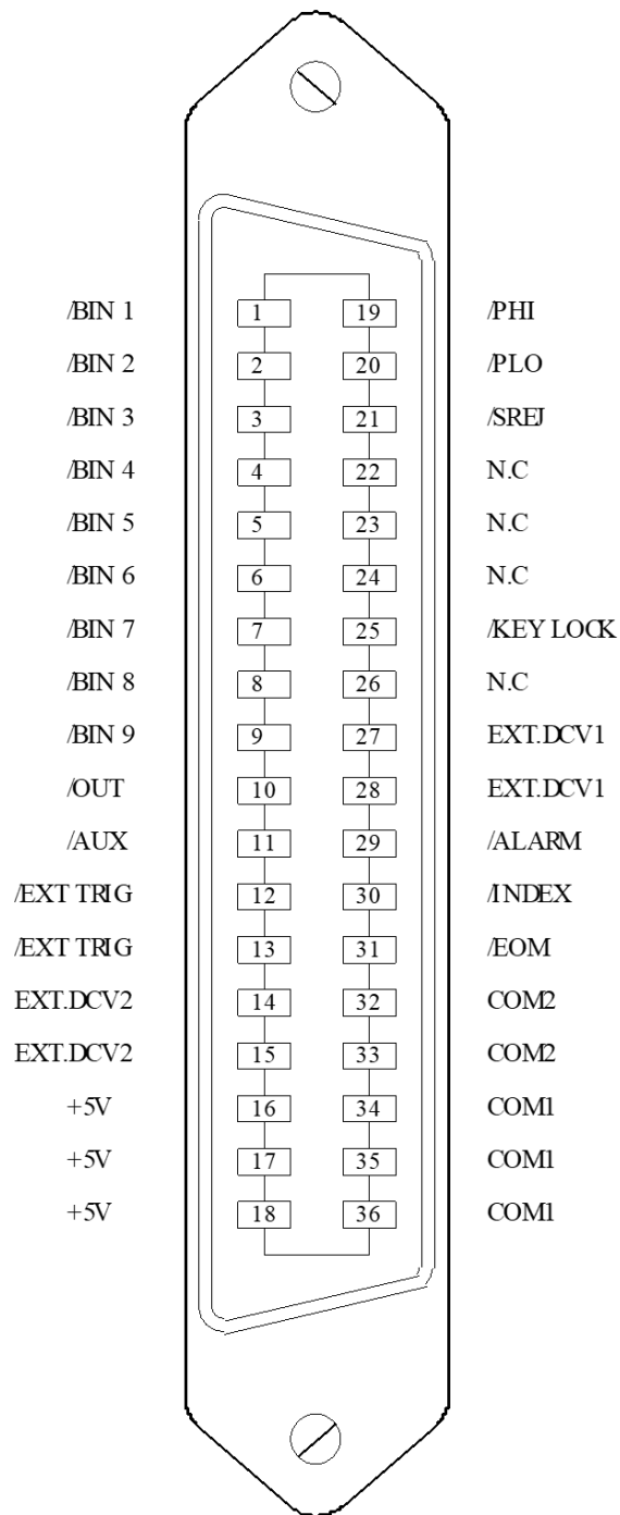
图 2 HANDLER 连接接口管脚定义
