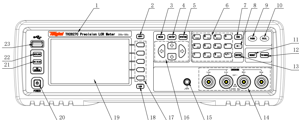
图 2-1. 前面板说明
