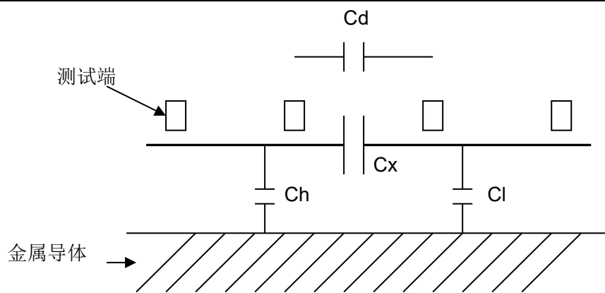
图 5-1 杂散电容的影响示意图
