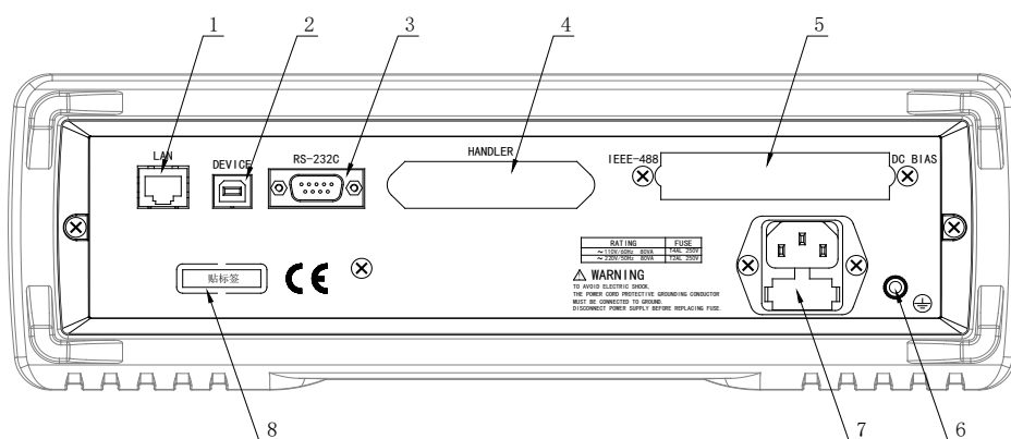
图 2-2. 后面板说明
