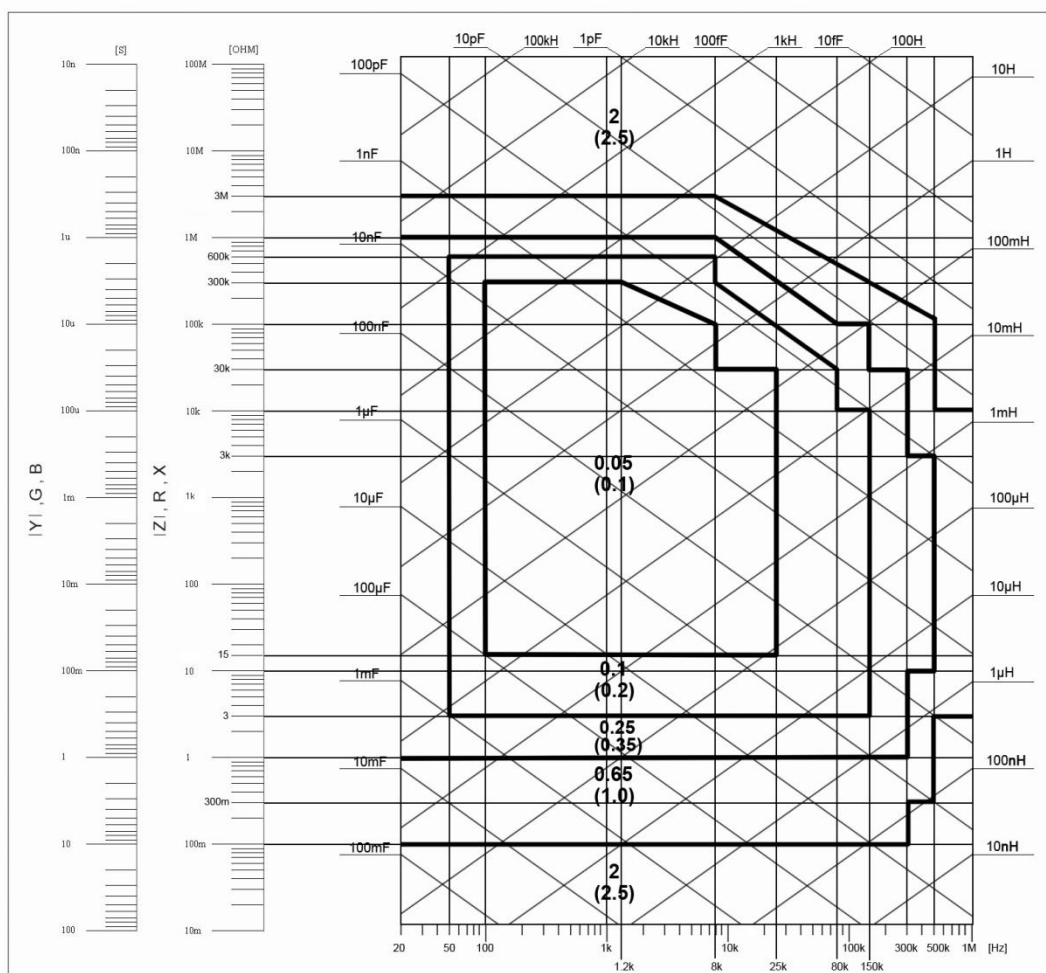
图 A 基本测量准确度 A
