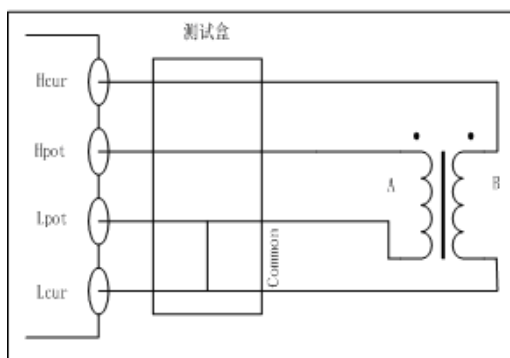
图 5—17 变压器测试连接示意图
