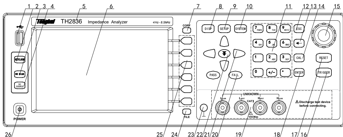
图 2-1 前面板说明
