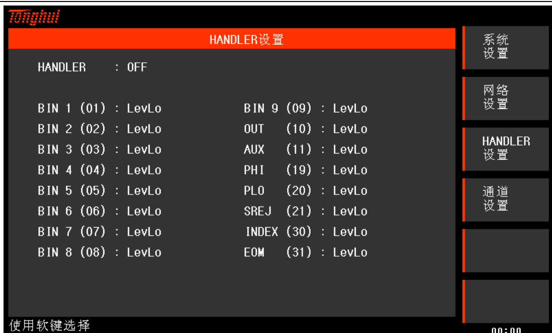
图 5-3 <HANDLER 设置>
