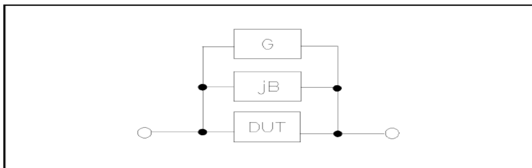
图 4-3 杂散导纳
