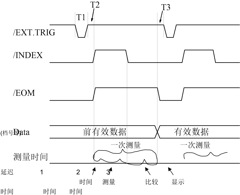
图 5-6 时序图
