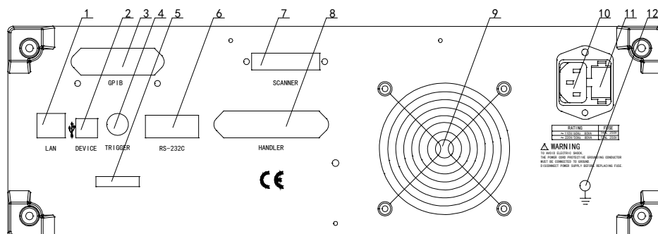
图 2-2 后面板说明
