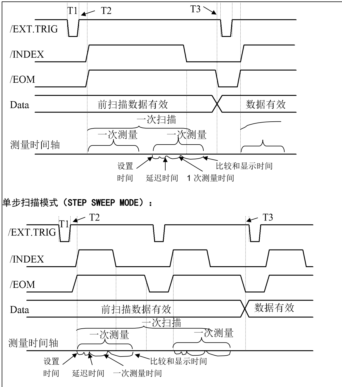
图 8-5 计时图解
