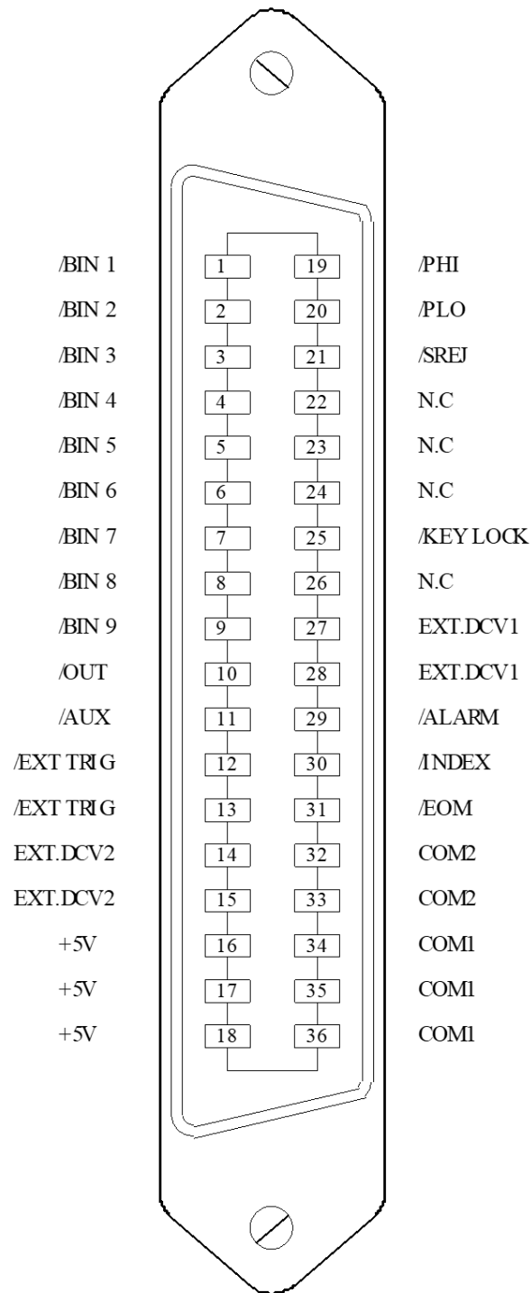
图 8-2 HANDLER 连接接口管脚定义
