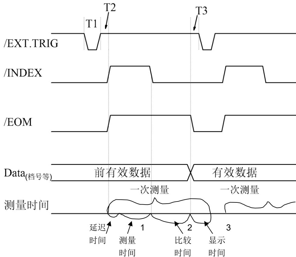
图 8-3 时序图
