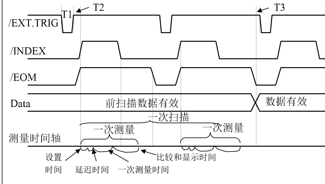
图 8-5 计时图解
