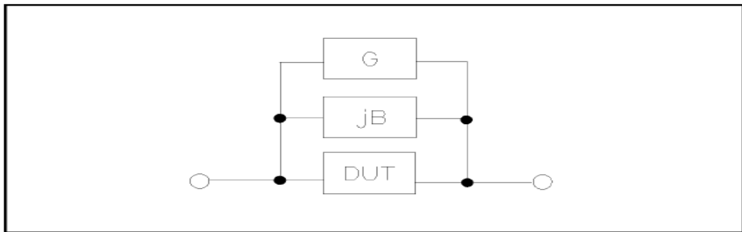
图 3-1 杂散导纳
