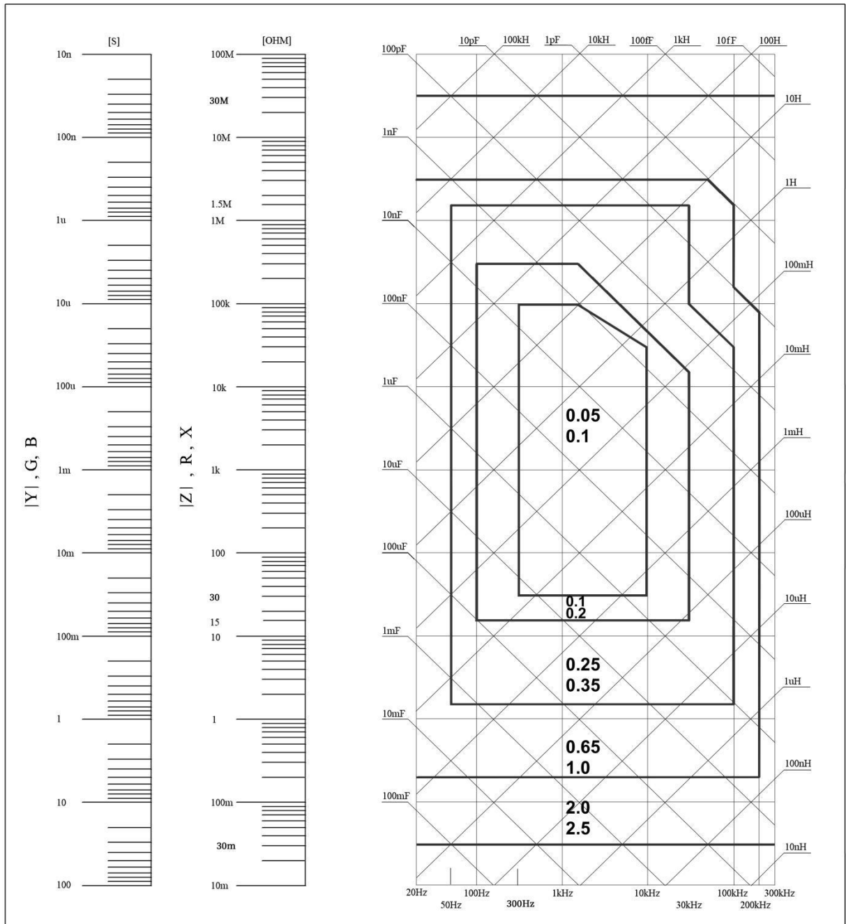
图 A 基本测量准确度 A
