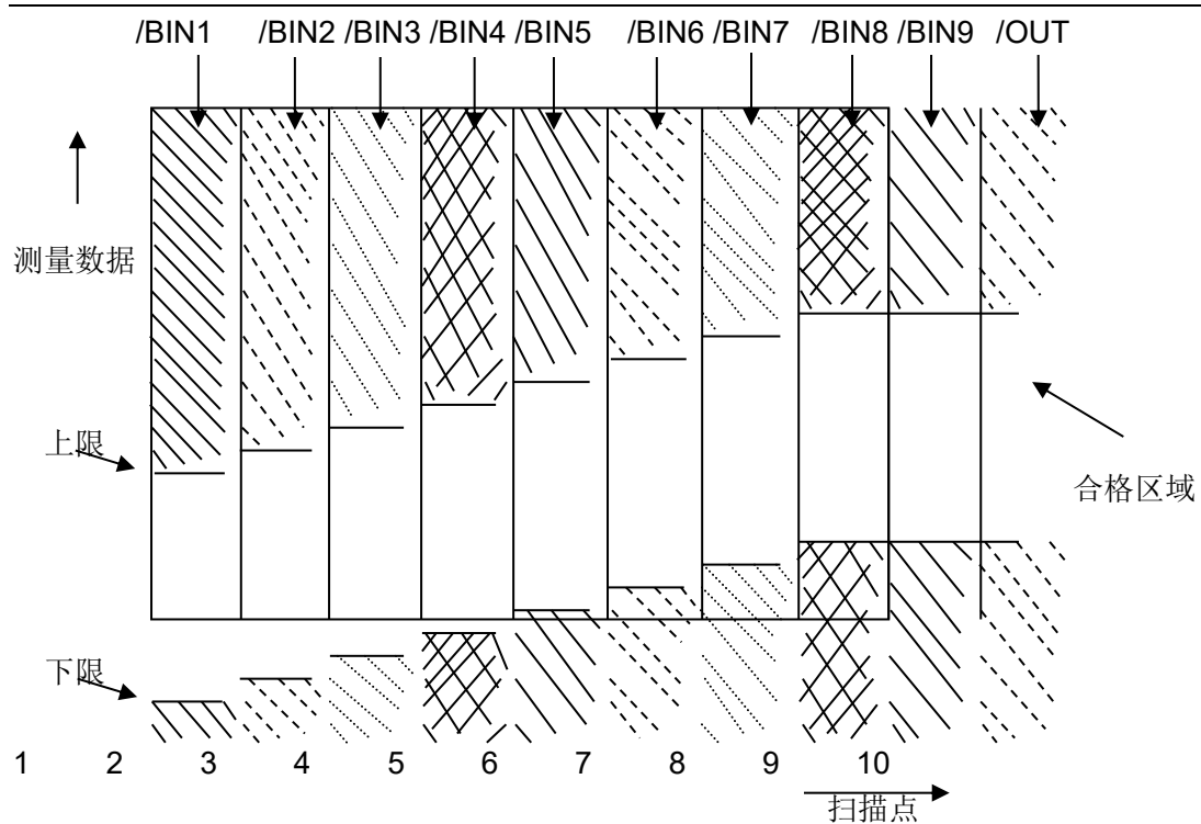
图 8-4 列表扫描比较功能信号区域示例
