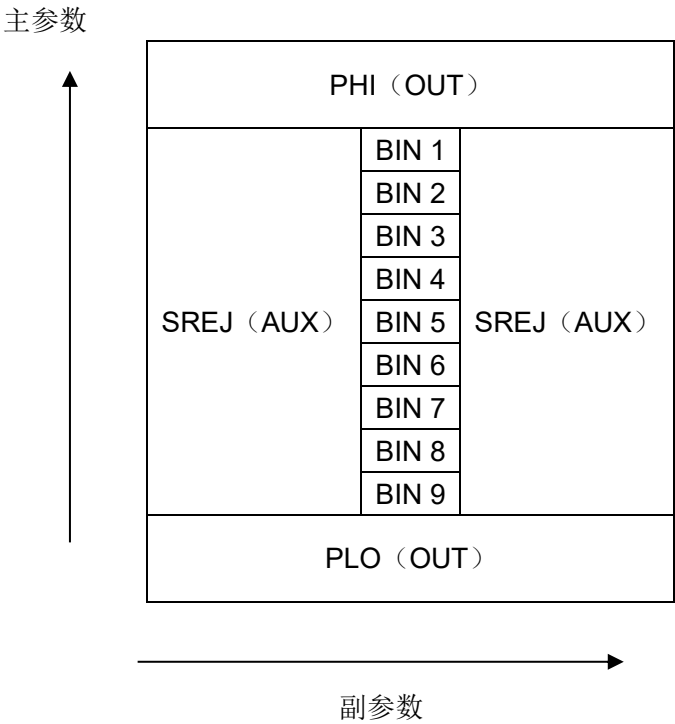
图 8-1 档比较功能/PHI, /PLO, /SREJ 信号的分配区域示例
