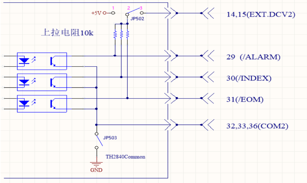
图 10-4 控制信号输出电路
