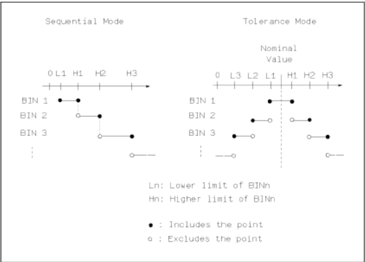
图 3-5-2 容差方式和连续方式
