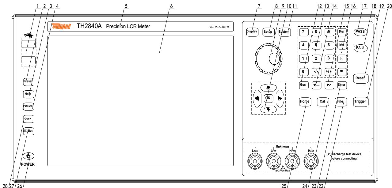
图 2-1. 前面板说明
