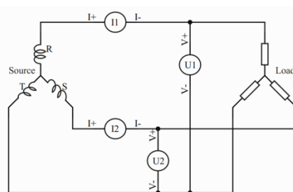
图 8-5 3P3W 示意图
