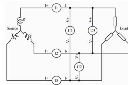
图 8-7 3V3A 示意图
