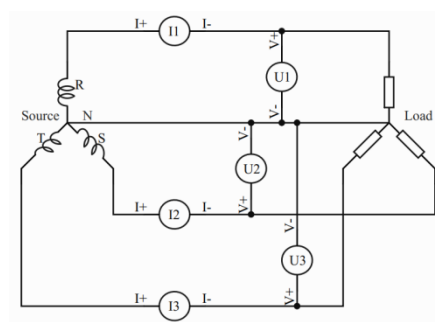
图 8-6 3P4W 示意图
