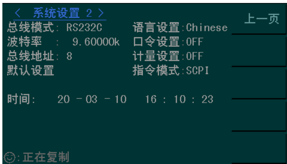
图 4.2.3.1 SYSTEM2 界面
