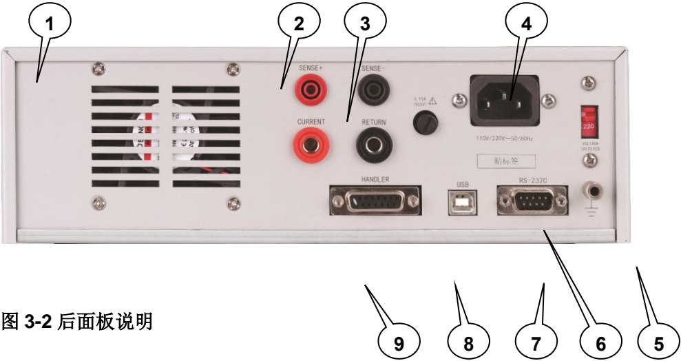
图 3-2 对 TH9410A/TH9411A 后面板进行了简要说明。
