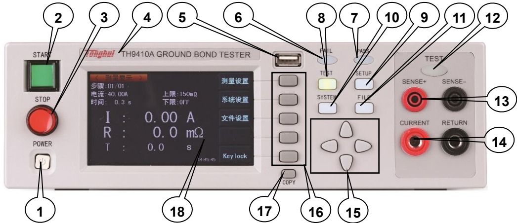
图 3-1 前面板说明
