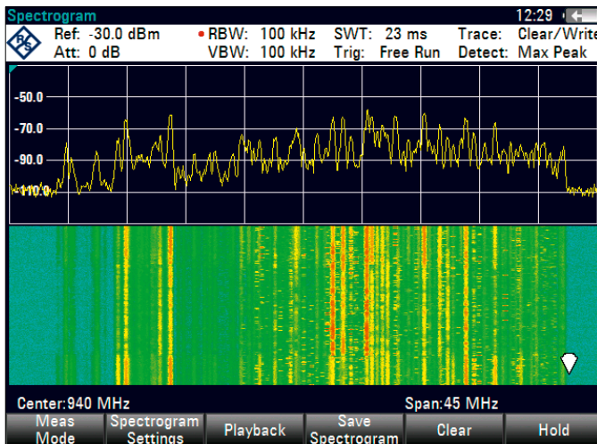
同时显示频谱和瀑布图
