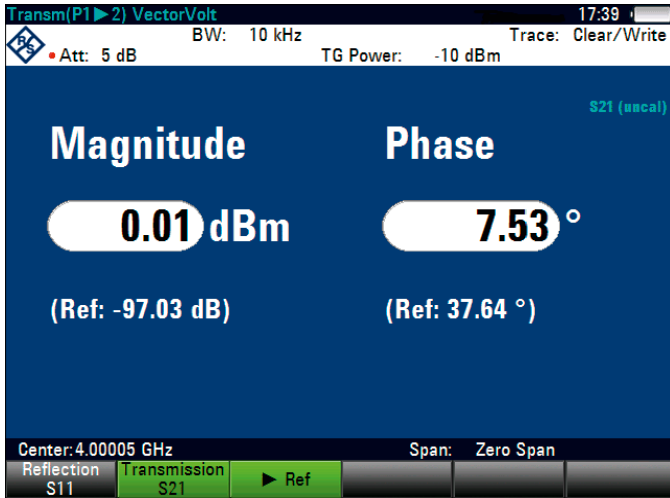
矢量电压表显示屏
