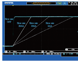
电流调节率
