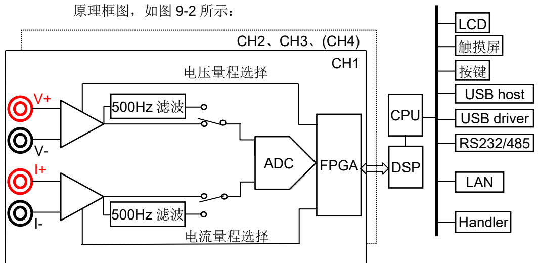
(图 9-2 原理框图)
