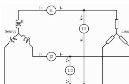
图 8-5 3P3W 示意图
