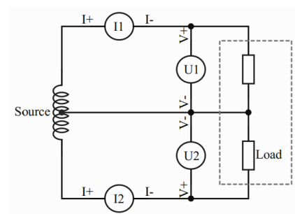
图 8-4 1P3W 示意图
