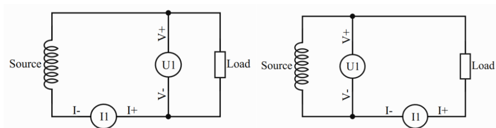
图 8-3 电流表外接(左)，电流表内接(右)—原理示意图
