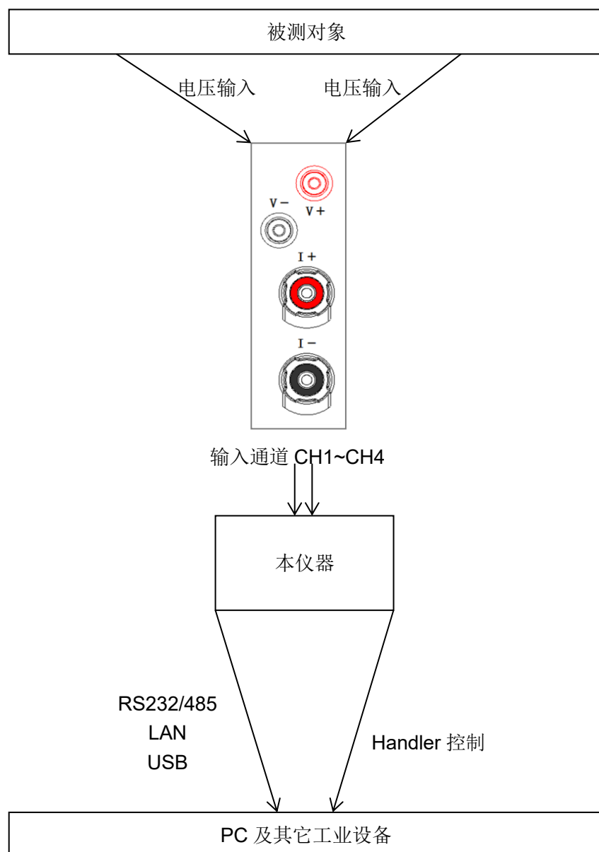
(图 9-1 系统构造)
