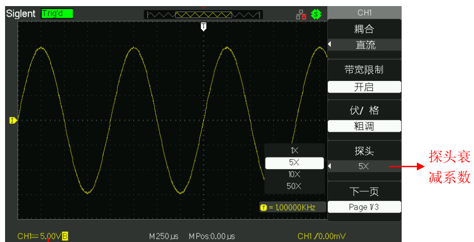
图 2-9 探头比例设置
