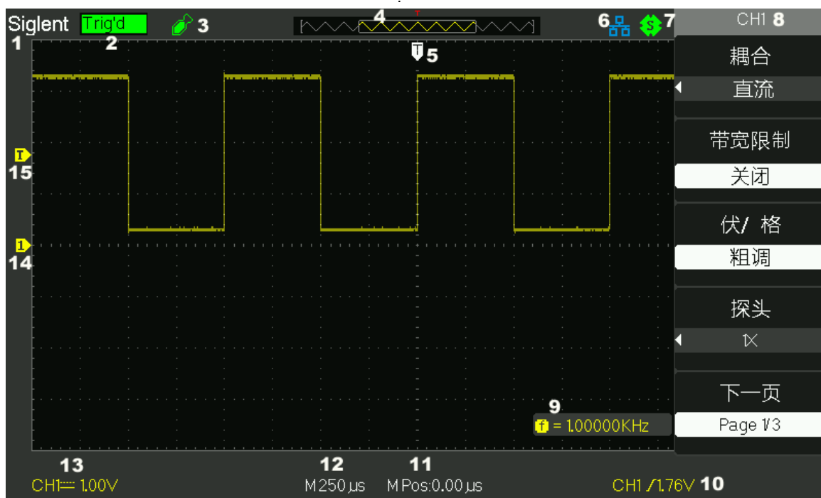
图 1-2 SDS1000A 界面显示区
