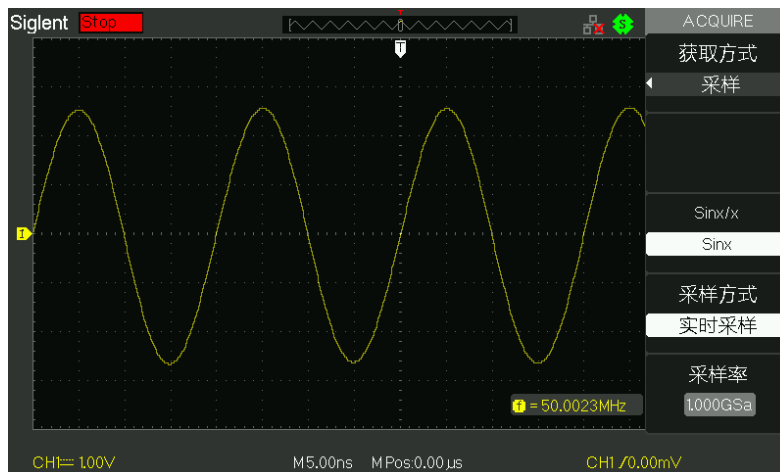
图 2-36 正弦插值
