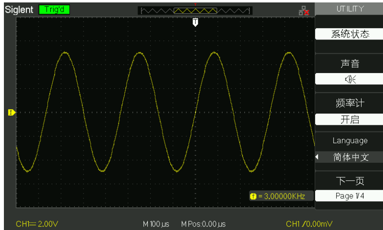
图 2-66 语言选择
