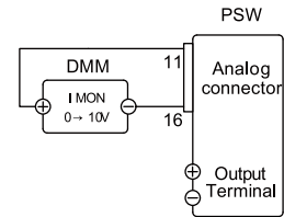
外部DMM监控输出电流
