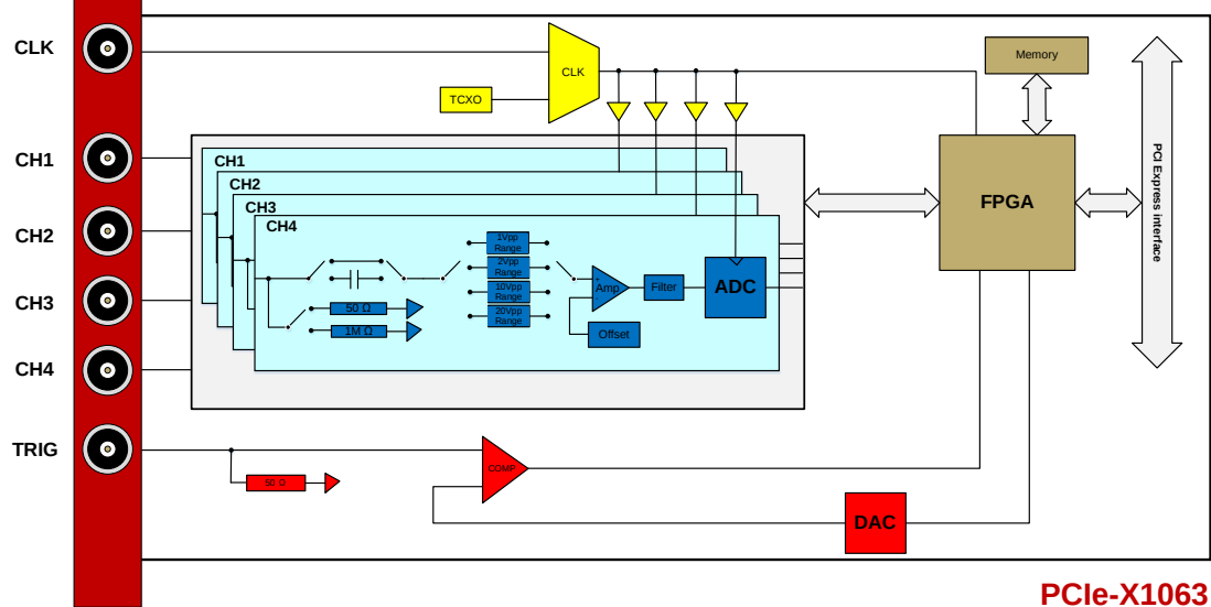
图 1 功能框图
