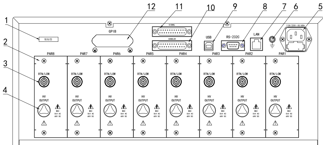
图 3-2 后面板说明
