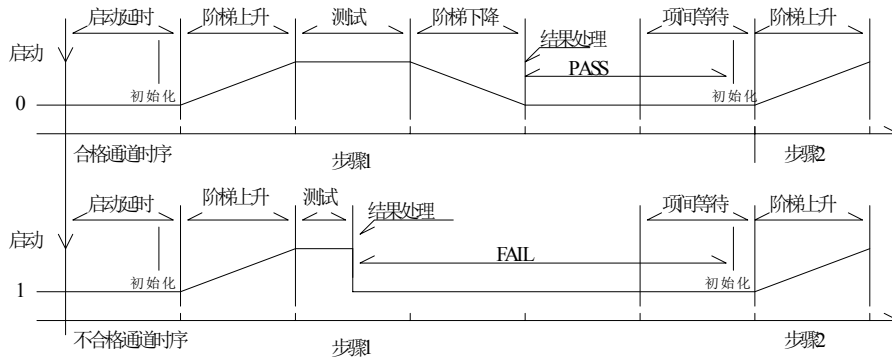
仪器测试时序示意图
