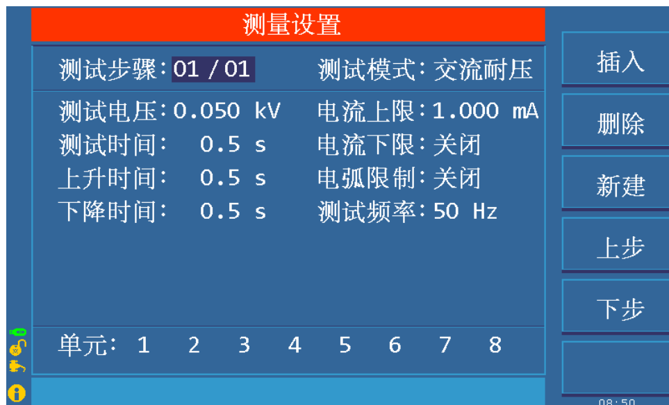
图 4.2.2 AC 设定界面示意
