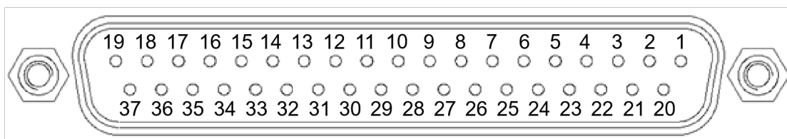
图 4-3-1 外部接口（EXT.I/O）示意图
