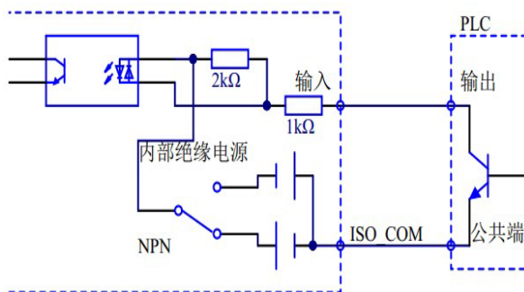
图 4-3-3-1.1 输入引脚 NPN 连接示意图
