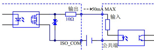
图 4-3-3-2.2 输出引脚负公共端连接示意图
